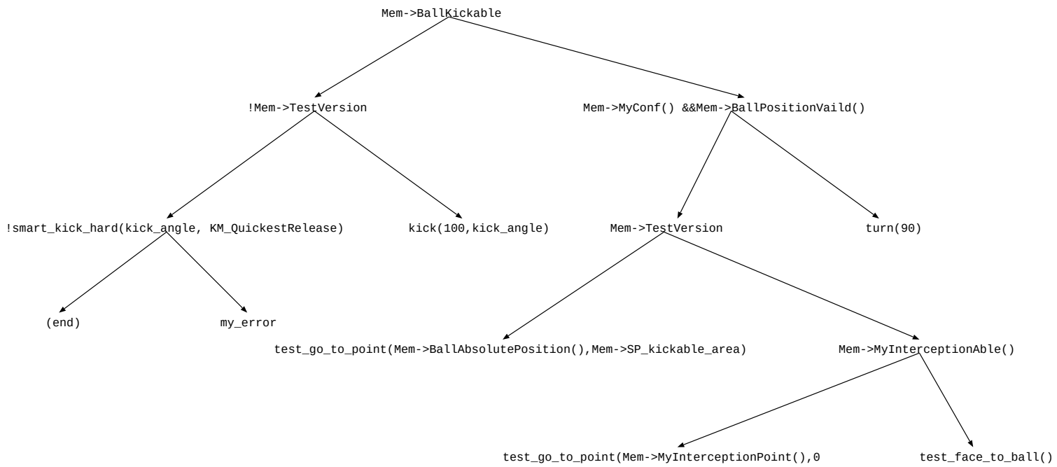
図 3.1: 初期アルゴリズム
