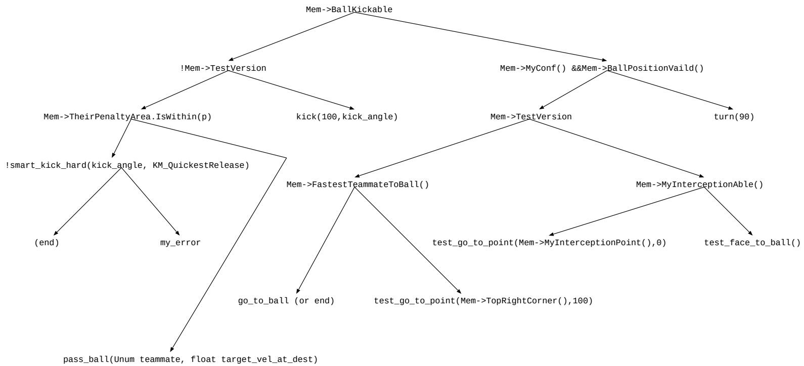
図 3.2: 実装アルゴリズム
