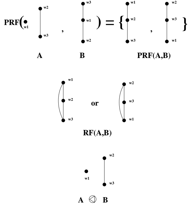
図 4 r_A の r_B によるリファインの集合とリファイン・オペレータの結果
