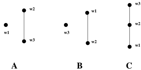
図 8 起源付きの選好関係によって誘発される順序付けが空である場合 .
