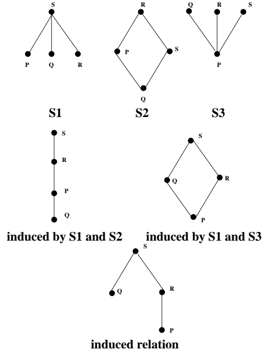
図 6 例 2.1 の形式化 .
