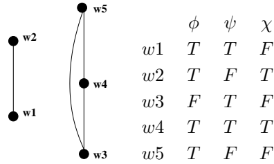
図 1 推論関係の解釈の例
