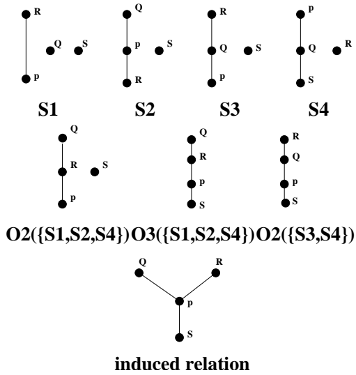
図 5 極大鎖による順序の例 .
