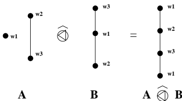
図 2 推移性に関わる例
