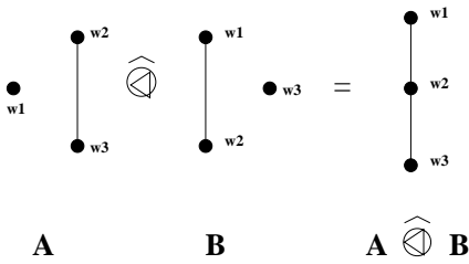
図 2 推移性に関わる例
