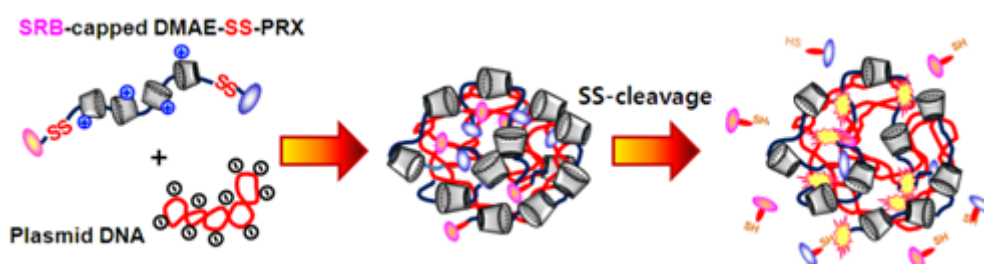
図1 ローダミンラベル化ポリロタキサン 1 によるSS結合に切断のイメージ
