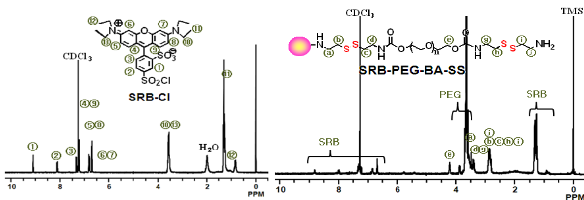
図 2 SRB-Clと(左)SRB-PEG-BA-SS(右)の ^1\text{H} NMR
