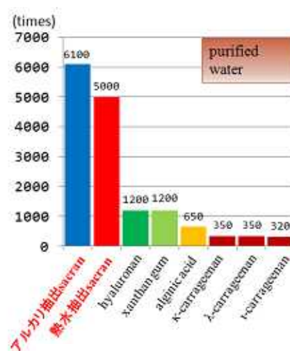
図1 純水における保水率
