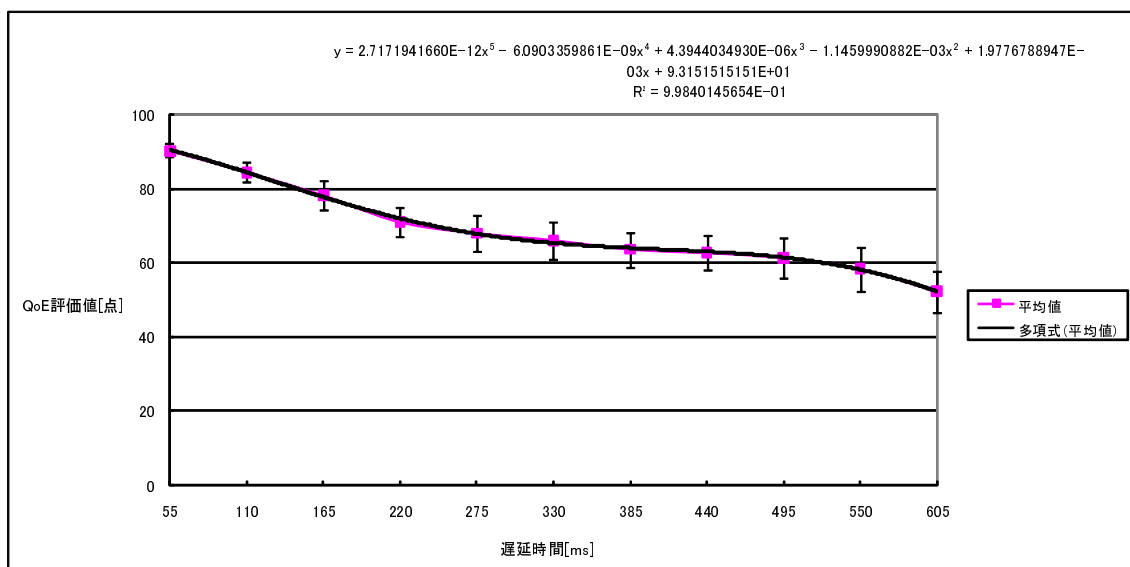
図 4.13: 本実験 2 のデータの五次回帰線
