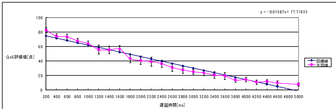
図 4.14: 本実験 2 のデータの単回帰線 2
