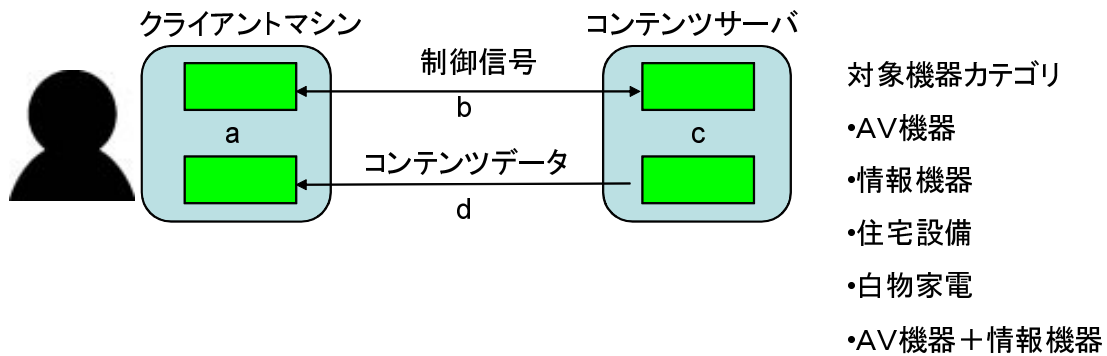
図 3.16: コンテンツ配信サービスモデル
