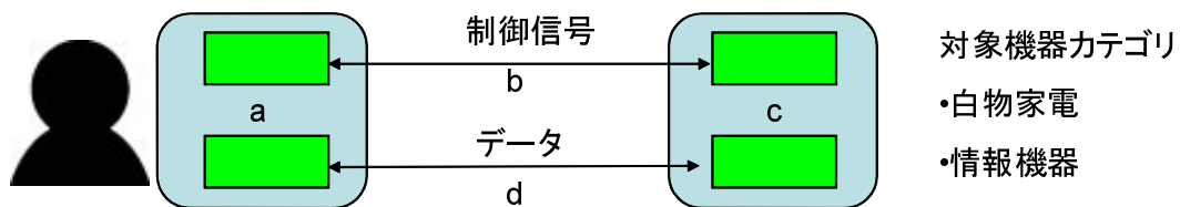
図 3.14: 機器の連動サービスモデル 3
