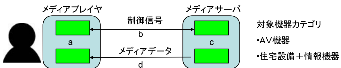
図 3.11: コンテンツ共有サービスモデル 2
