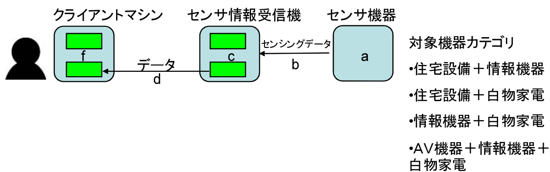
図 3.20: センサ情報の通知サービスモデル 2
