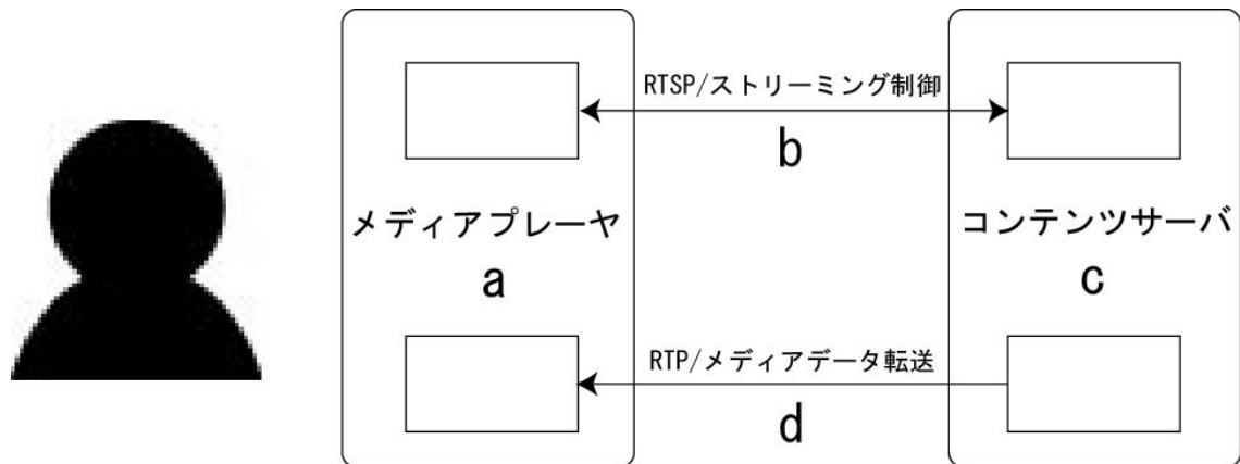
図 3.32: ストリーミングサービスモデル
