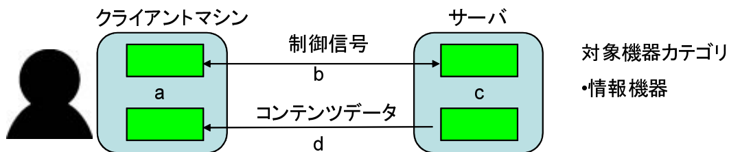
図 3.25: ネットゲームサービスモデル
