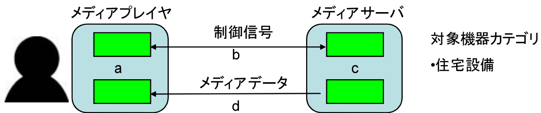
図 3.12: 機器の連動サービスモデル 1
