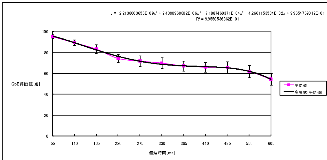
図 4.19: 本実験 2 の修正データの四次回帰線
