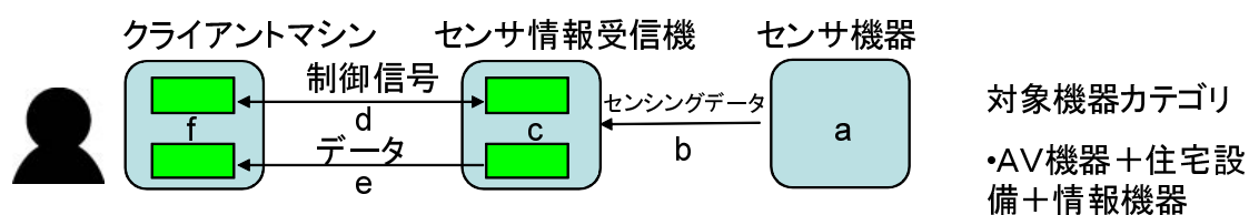
図 3.21: センサ情報の通知サービスモデル 3
