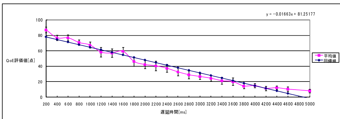
図 4.20: 本実験 2 の修正データの単回帰線 2
