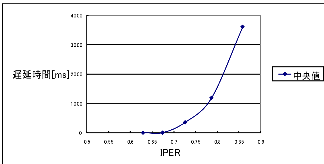
図 5.1: IPER と遅延時間の関係
