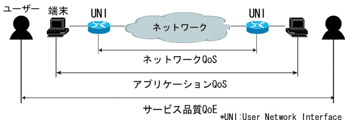
図 3.1: QoE と QoS の関係図
