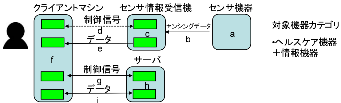
図 3.29: センサ情報の通知とコンテンツ配信の複合サービスモデル
