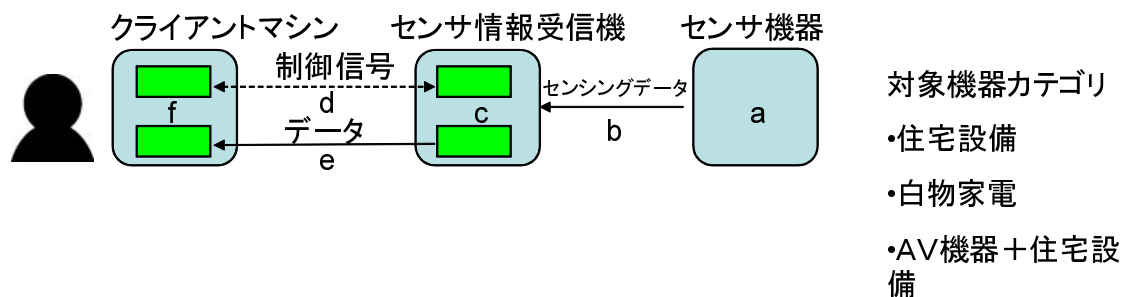
図 3.19: センサ情報の通知サービスモデル 1
