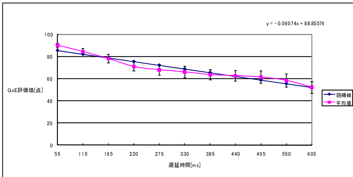
図 4.12: 本実験 2 のデータの単回帰線 1
