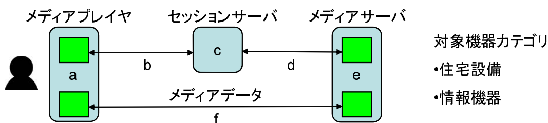
図 3.18: 通話サービスモデル
