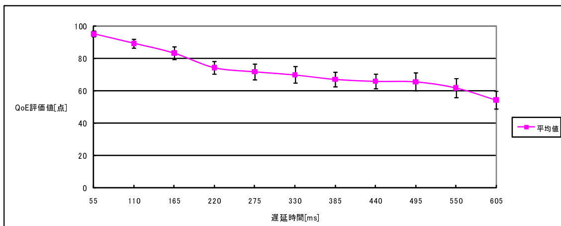
図 4.10: 本実験 2 のデータの平均値 1
