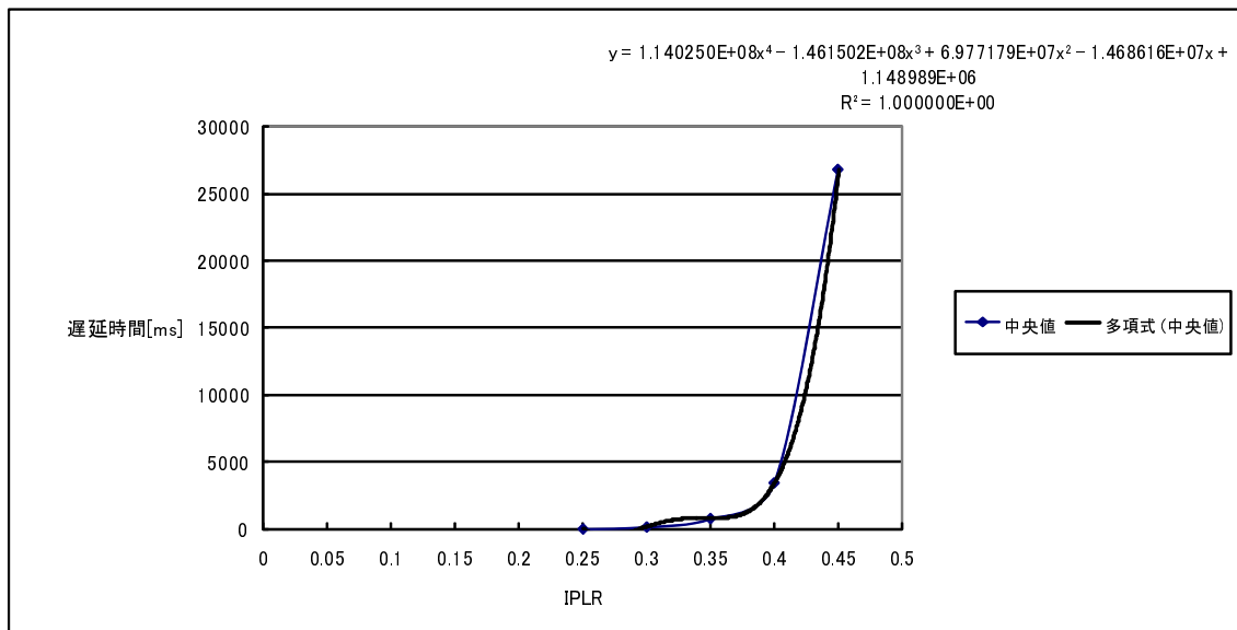
図 5.4: IPLR と遅延時間の関係と回帰線
