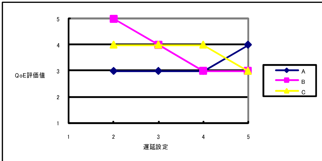
図 4.22: データの単回帰線の評価結果 1
