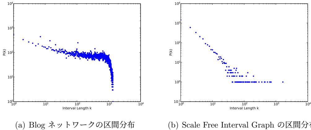
図 3.4: 区間分布
