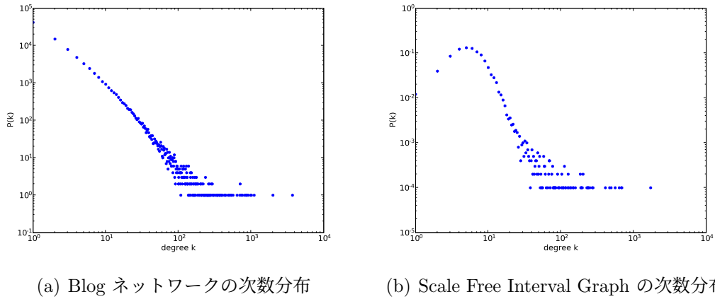
図 3.5: 次数分布
