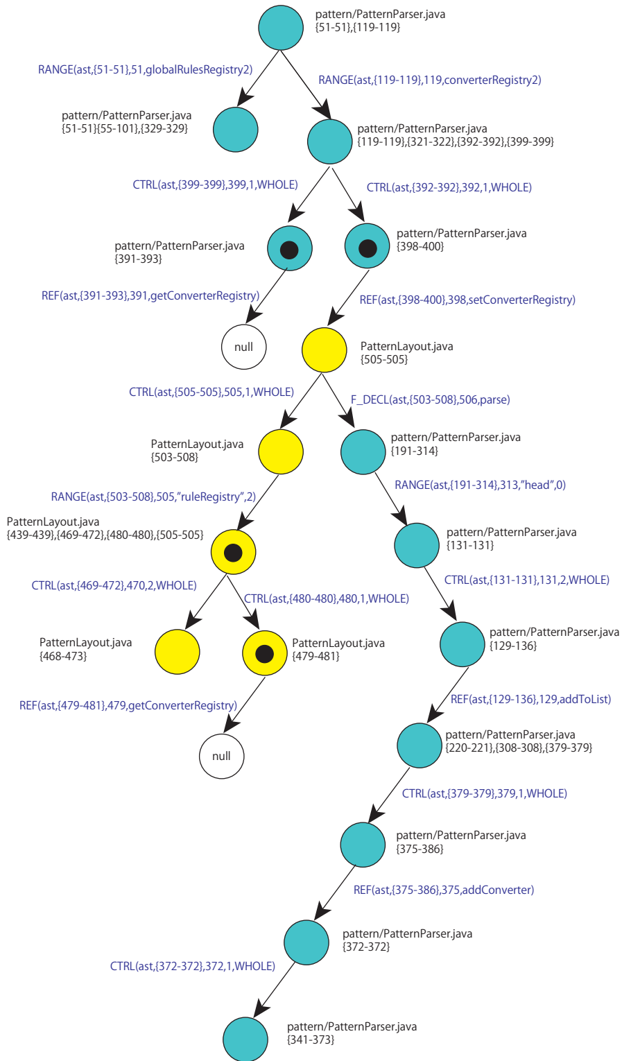
図 5.9: ナビゲーション木の生成過程
