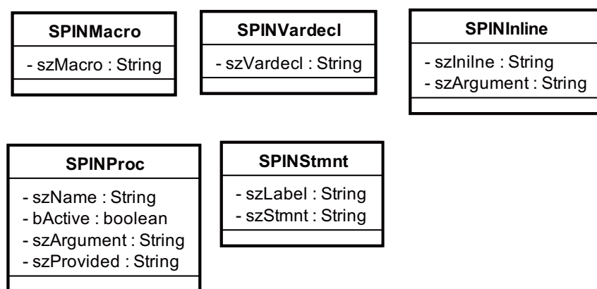
図 5.6: SPINCode の属性
