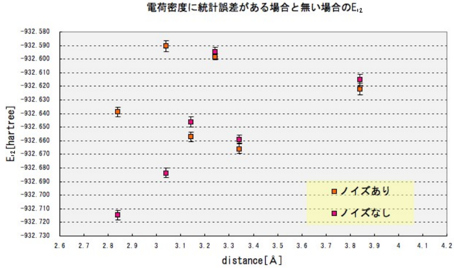
図 5.0.7: 電荷密度に統計誤差を含む場合と含まない場合の E_{12}
