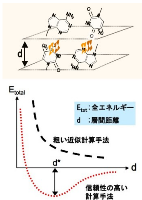
図 2.5.2: 塩基間距離依存性を示すエネルギー
