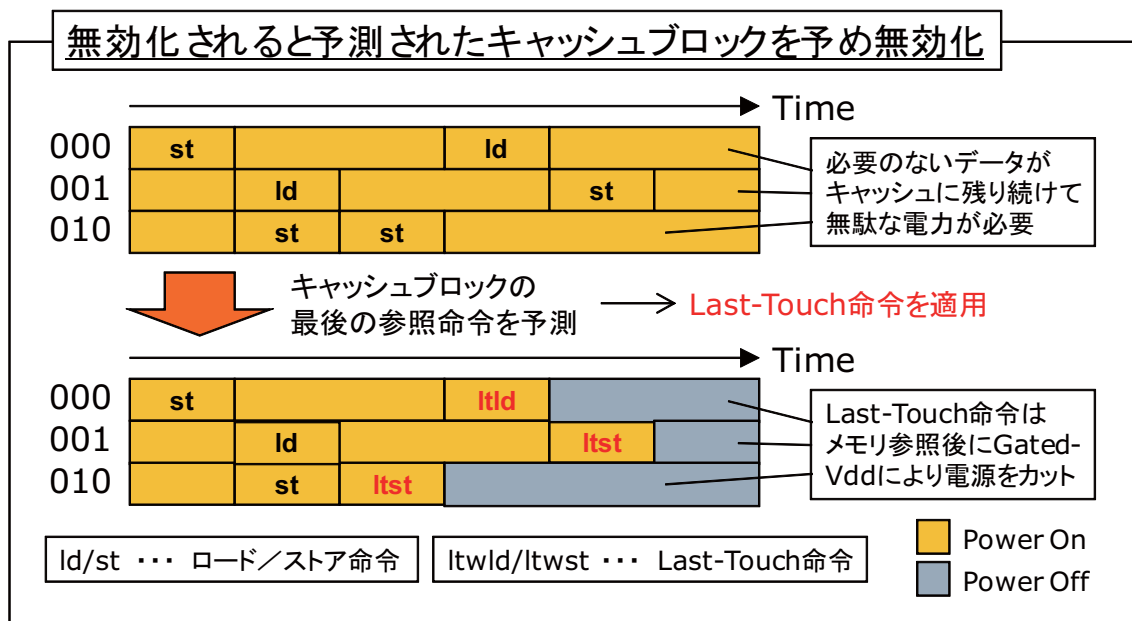
図 2.4: ソフトウェア Self-Invalidation による電力制御
