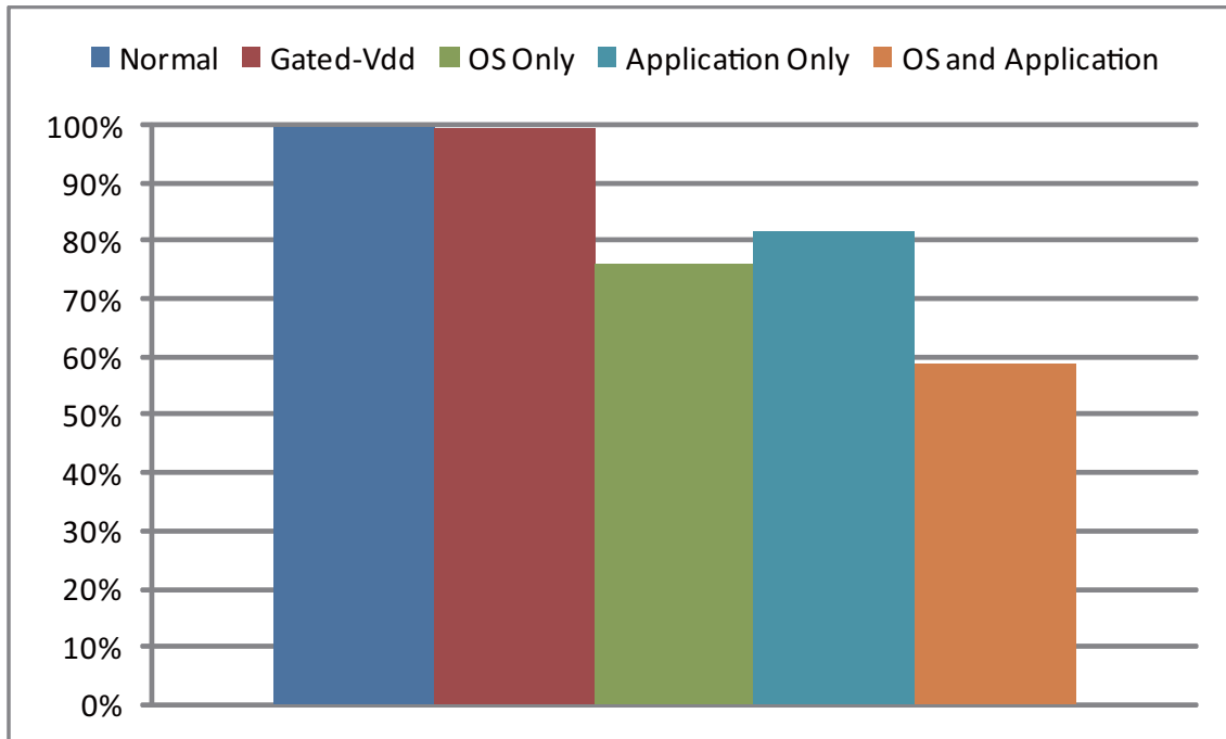
図 5.2: 計測 2 における 5 つの実行状態の消費電力
