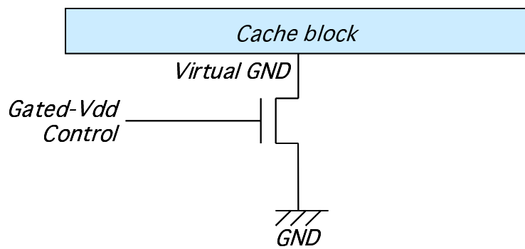
図 2.2: キャッシュブロック単位での電圧制御の例
