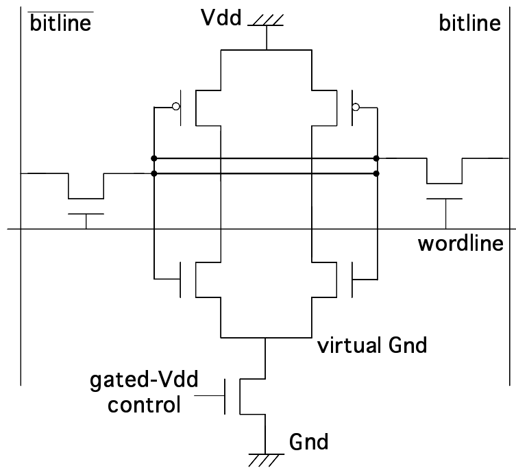
図 2.1: NMOS トランジスタによる SRAM セルの gated-Vdd 構成
