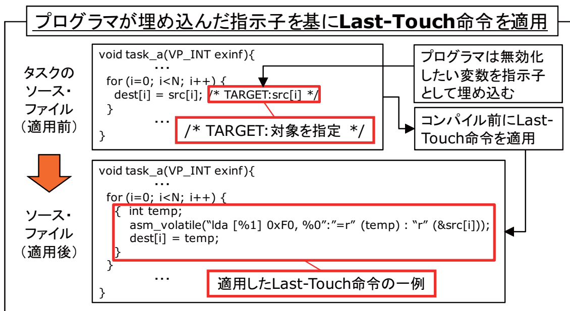
図 4.2: プログラマによる Last-Touch 命令の適用例
