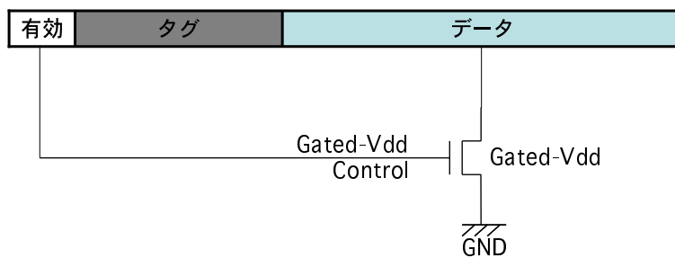
図 3.3: キャッシュメモリの供給電力制御
