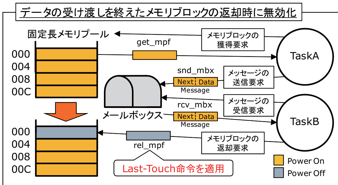
図 4.1: メールボックスと固定長メモリプールの処理での Last-Touch 命令の適用例
