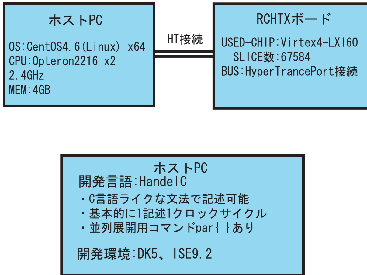
図 4.12: ハードウェアの実験環境
