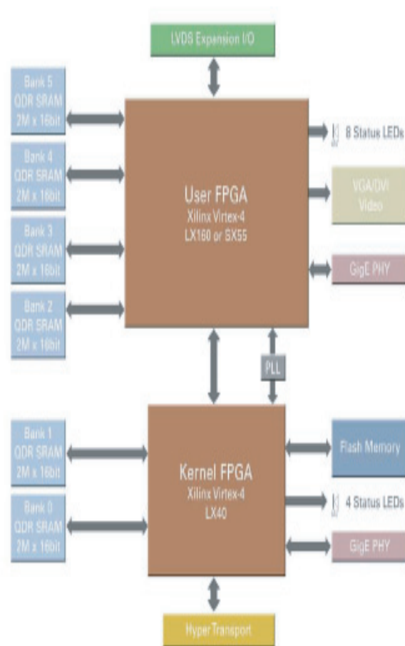
図 4.13: RCHTX ボード概略図
