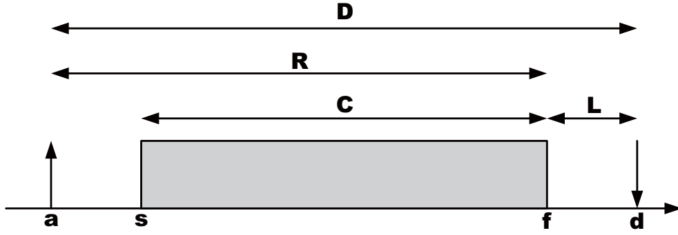
図 4.2: タスクの時間情報
