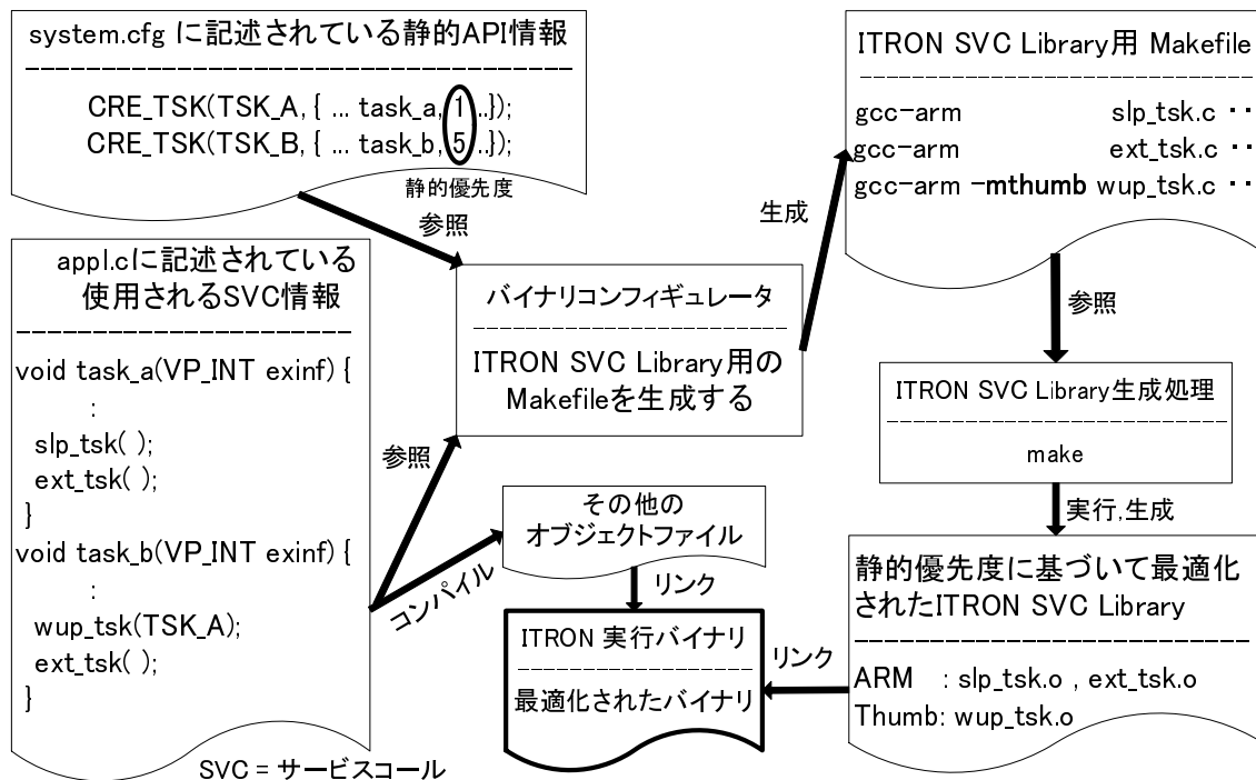
図 3.3: サービスコールライブラリに対するコンフィギュレーションの概要
