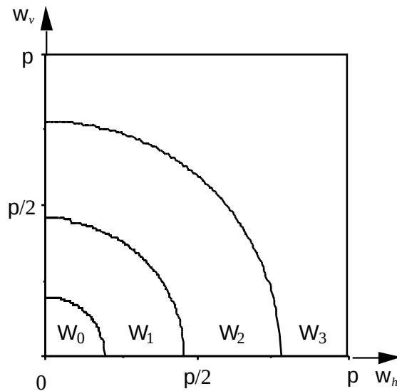
図 4.1 最適帯域分割パターン（水平・垂直相関非分離型画像モデル， r=0.9 ， M=4 ）
