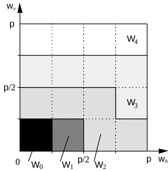
図 4.15 帯域ブロックをベースとする適応帯域分割パターン ( 画像 "Lenna" , M=5 , N^2=16 )
