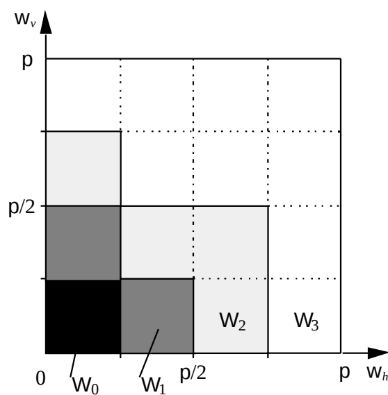
図 4.10 帯域ブロックをベースとする適応帯域分割パターン （画像 "Hada" , M=4 , N^2=16 ）
