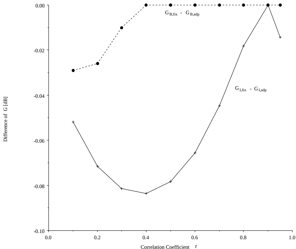
図 4.7 固定の最適帯域分割に対する量子化雑音改善量 G の変化 ( M=4 ) (パラメータ：相関係数値 r )
