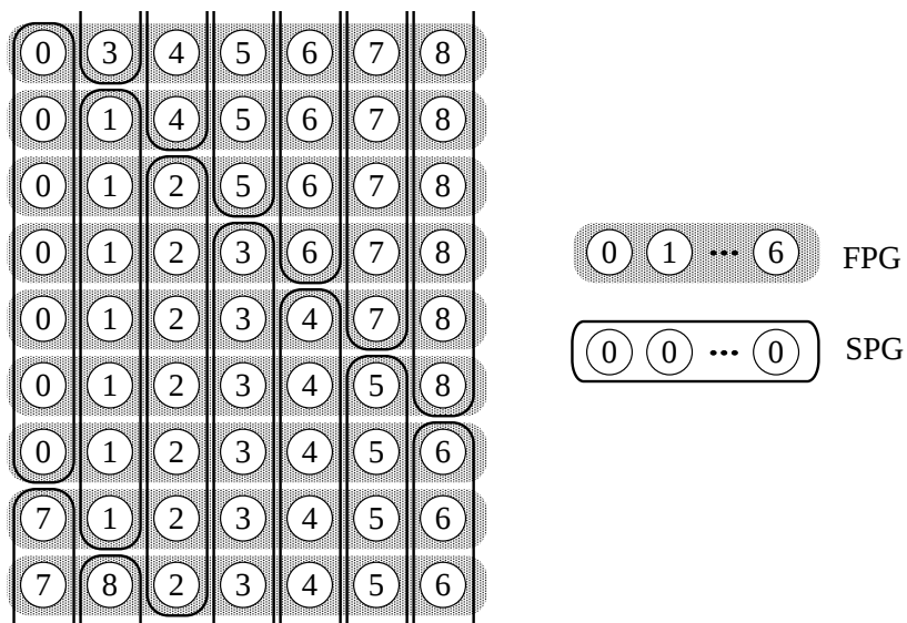
図 4.11: ノード数 63 の構成の行列表現 (7 ノード/パリティグループ)
