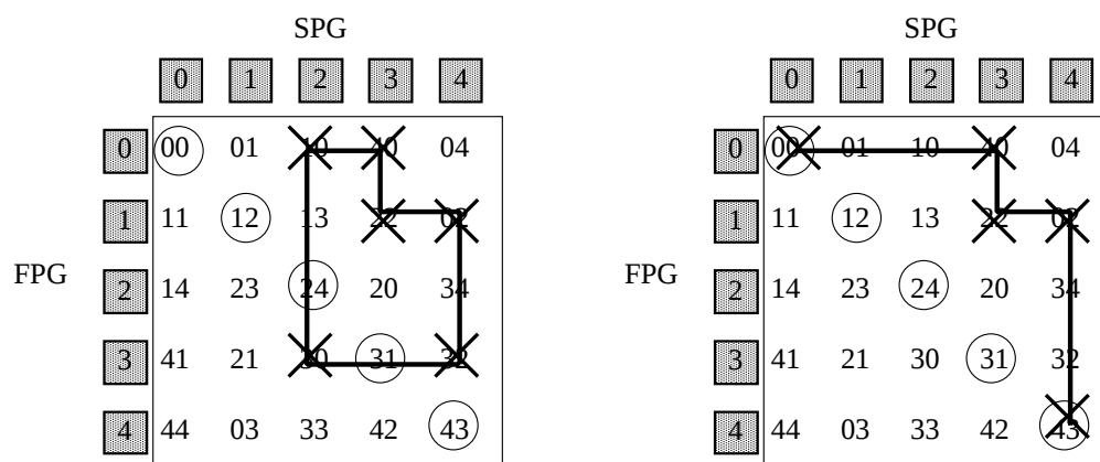
図 4.6: マスクできない故障パタンの例
