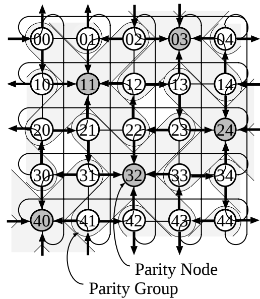
図 3.4: SPG(Second Parity Groups) の構成
