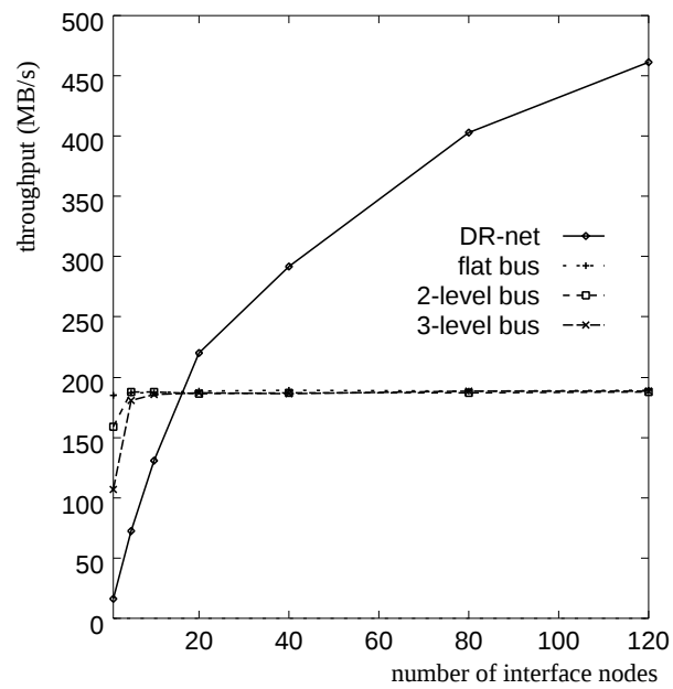
図 6.9: 読み出しのスループット (ディスクノード数=1,000)
