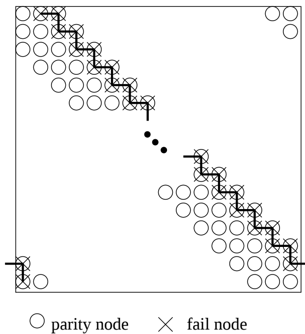
図 4.7: マスク可能な故障パターン (パリティ固定)
