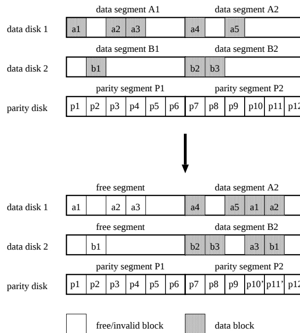
図 7.2: セグメントクリーニング
