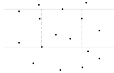
図 3.11: 下辺が左边を決める場合
