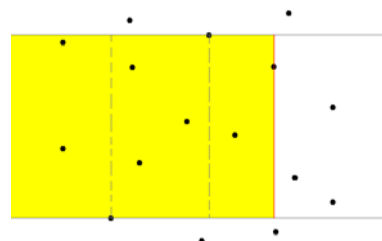
図 3.6: 右辺候補のディスクレパンシー
