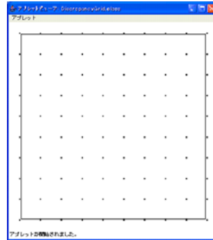
図 2.14: 点をすべて含む最も小さい長方形を少し小さくした場合
