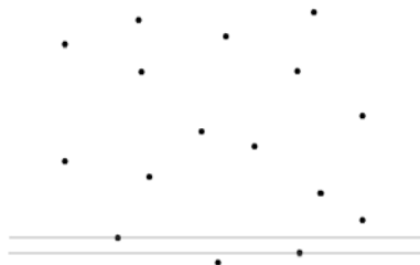
図 3.3: 上辺が一番上までいった後
