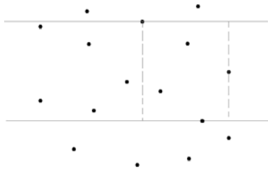
図 3.10: 上辺が左边を決める場合
