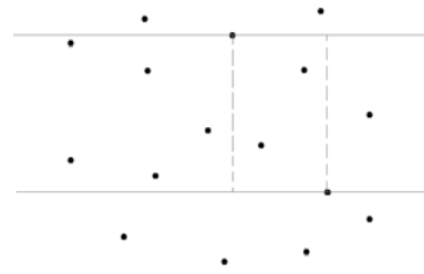
図 3.9: 上辺が左边を決める場合
