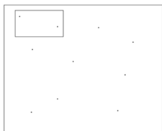
図 1.3: 四角形を考慮する方法
