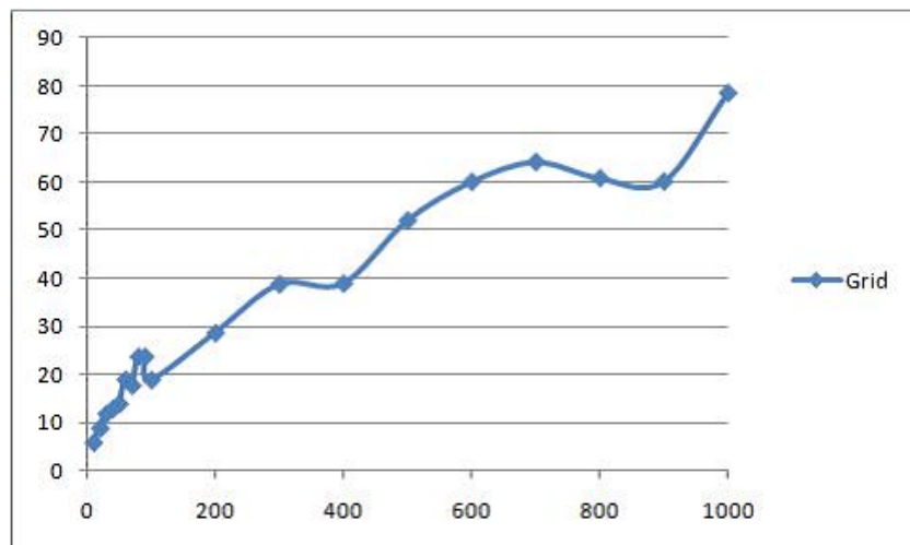
図 4.15: 格子状点集合における点数とディスクリパンシーの関係
