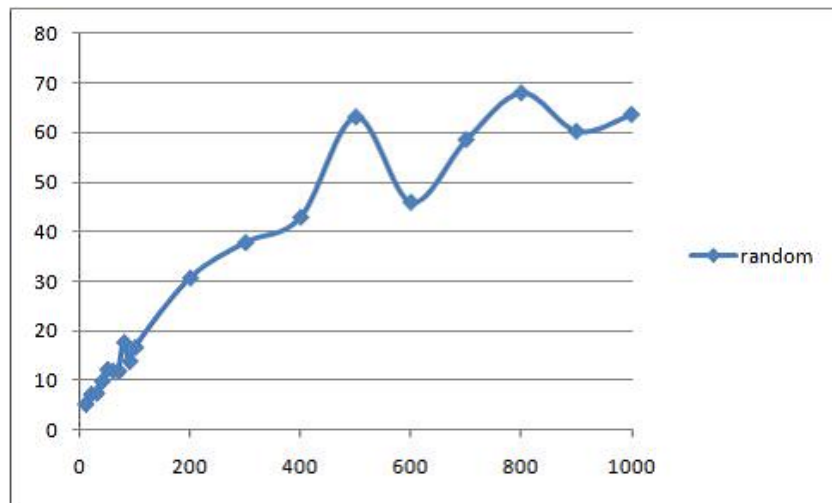
図 4.14: ランダム点集合における点数とディスクリパンシーの関係
