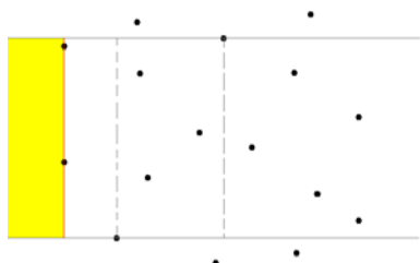
図 3.5: 左辺候補のディスクレパンシー
