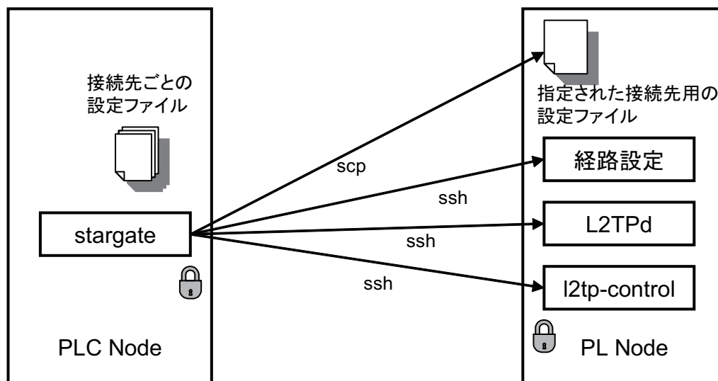
図 6.13: SSH を用いたトンネル接続の実行
