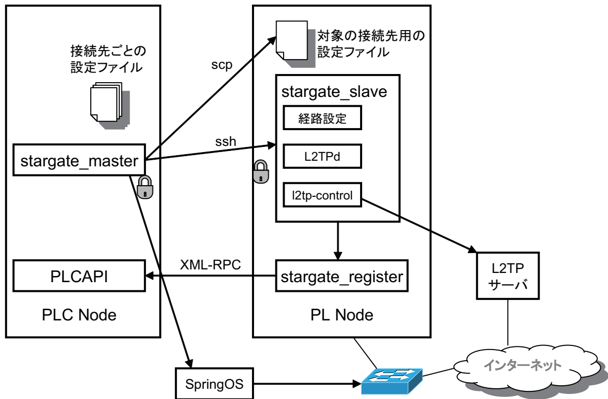
図 6.14: 3 分割構成
