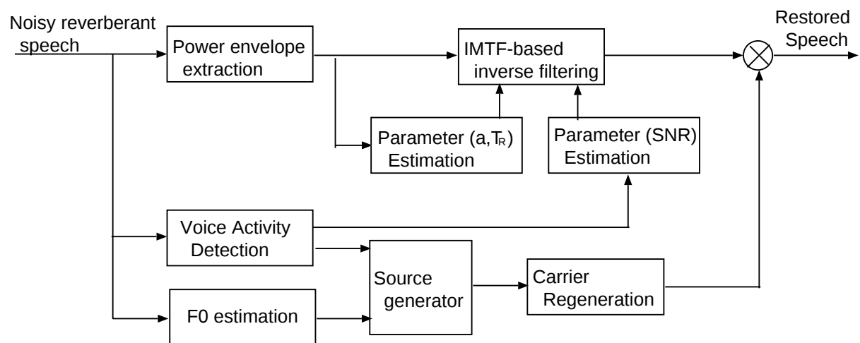
図 5.2: 音声明瞭度と聴き取りにくさを改善する雑音残響除去法の概要
