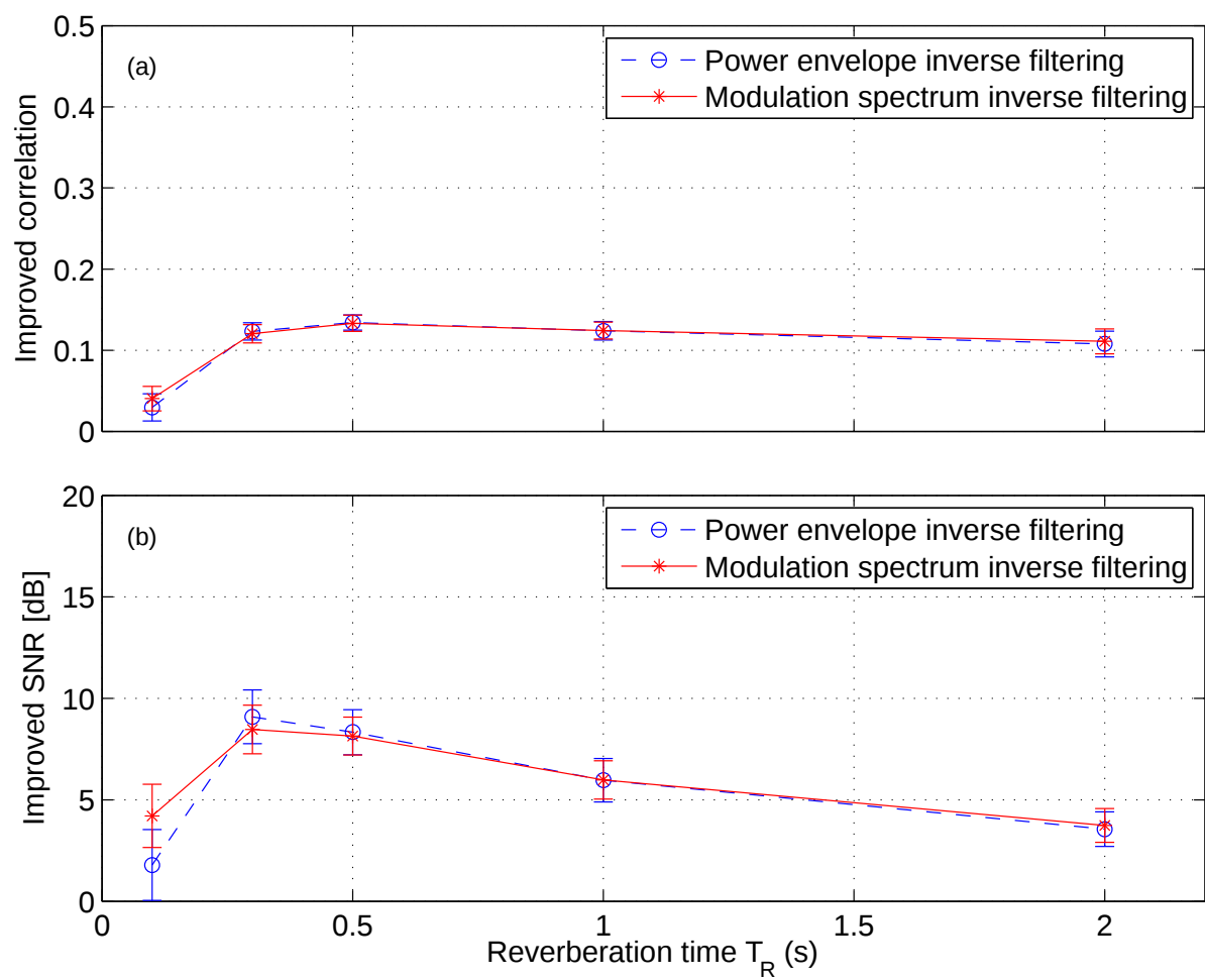
図 6.5: 帯域制限雑音で構成されるパワーエンベロープの評価結果：(a) Correlation と (b) SNR の改善度
