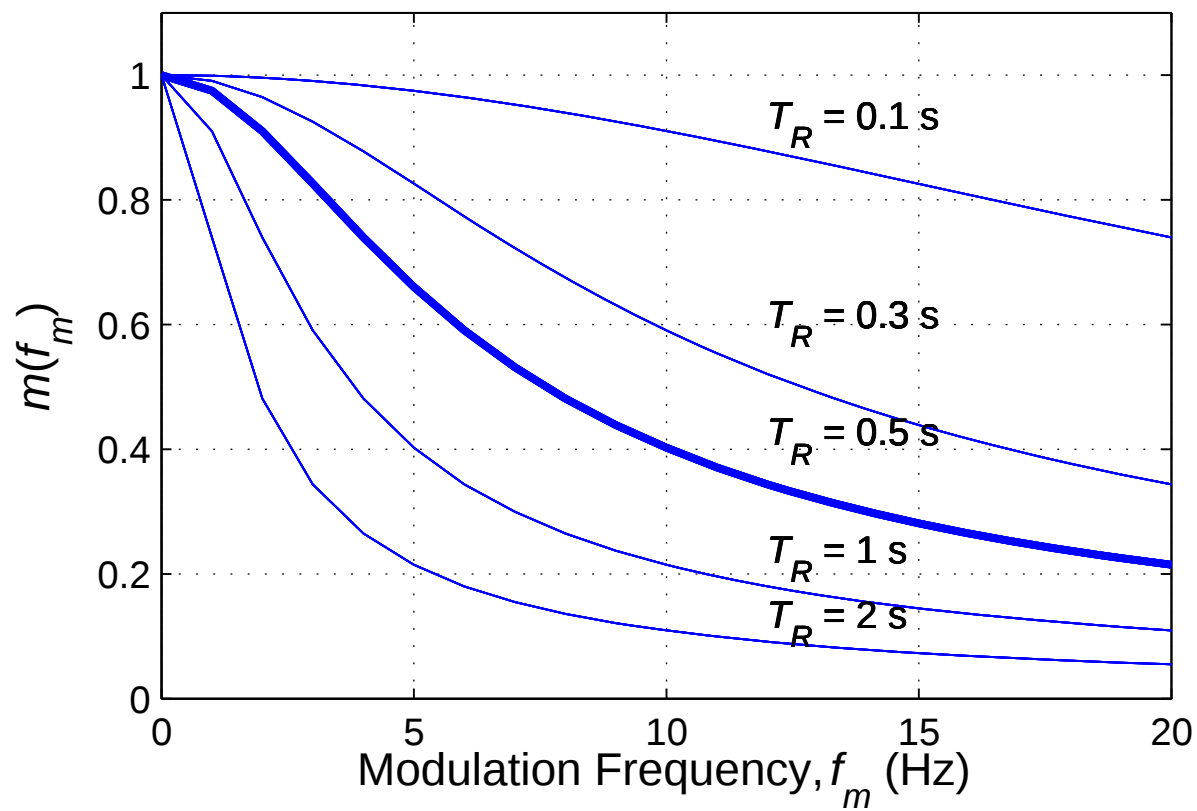
図 4.2: 残響環境での MTF m(f_m) の特性
