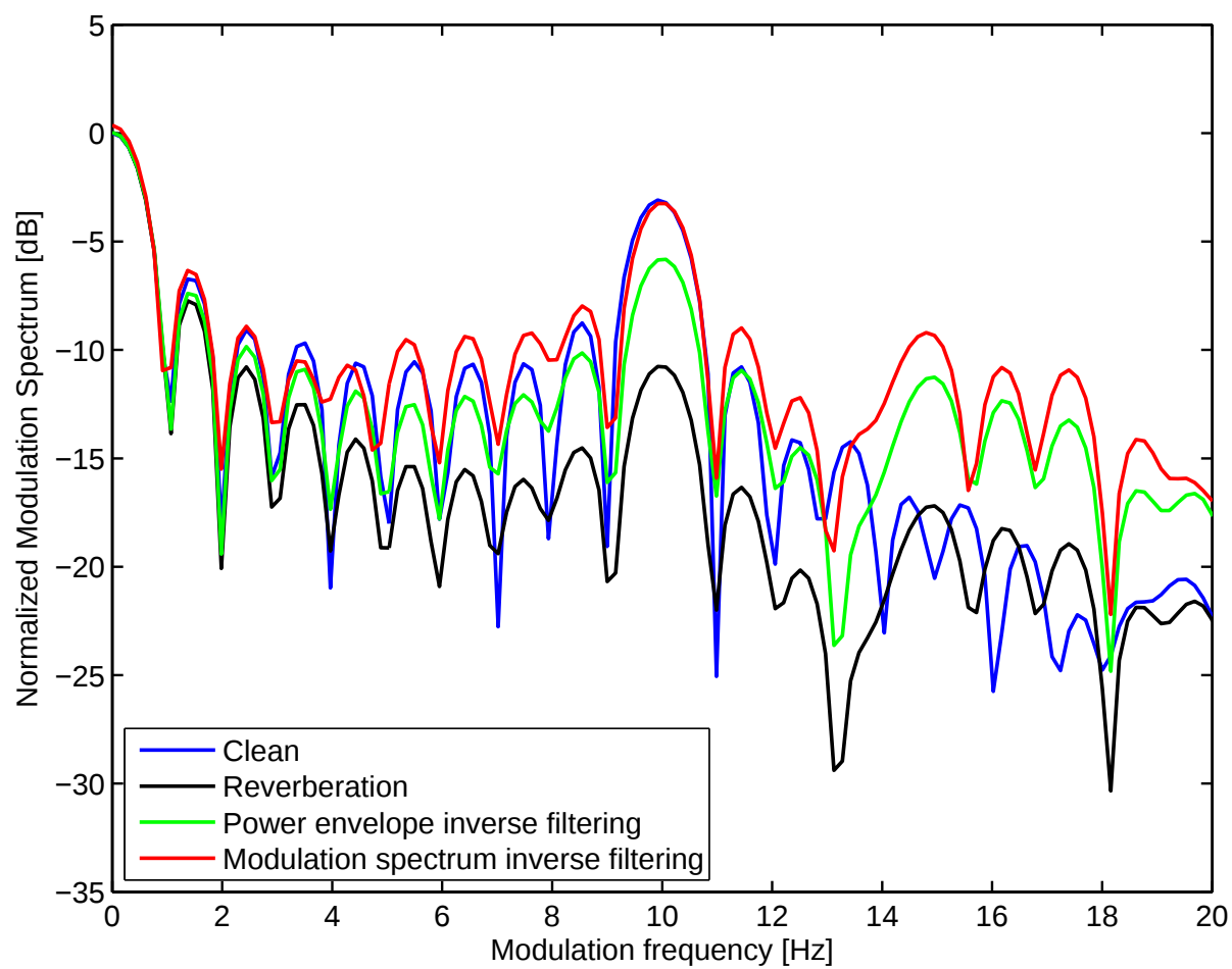
図 6.2: 正弦波信号の変調スペクトル
