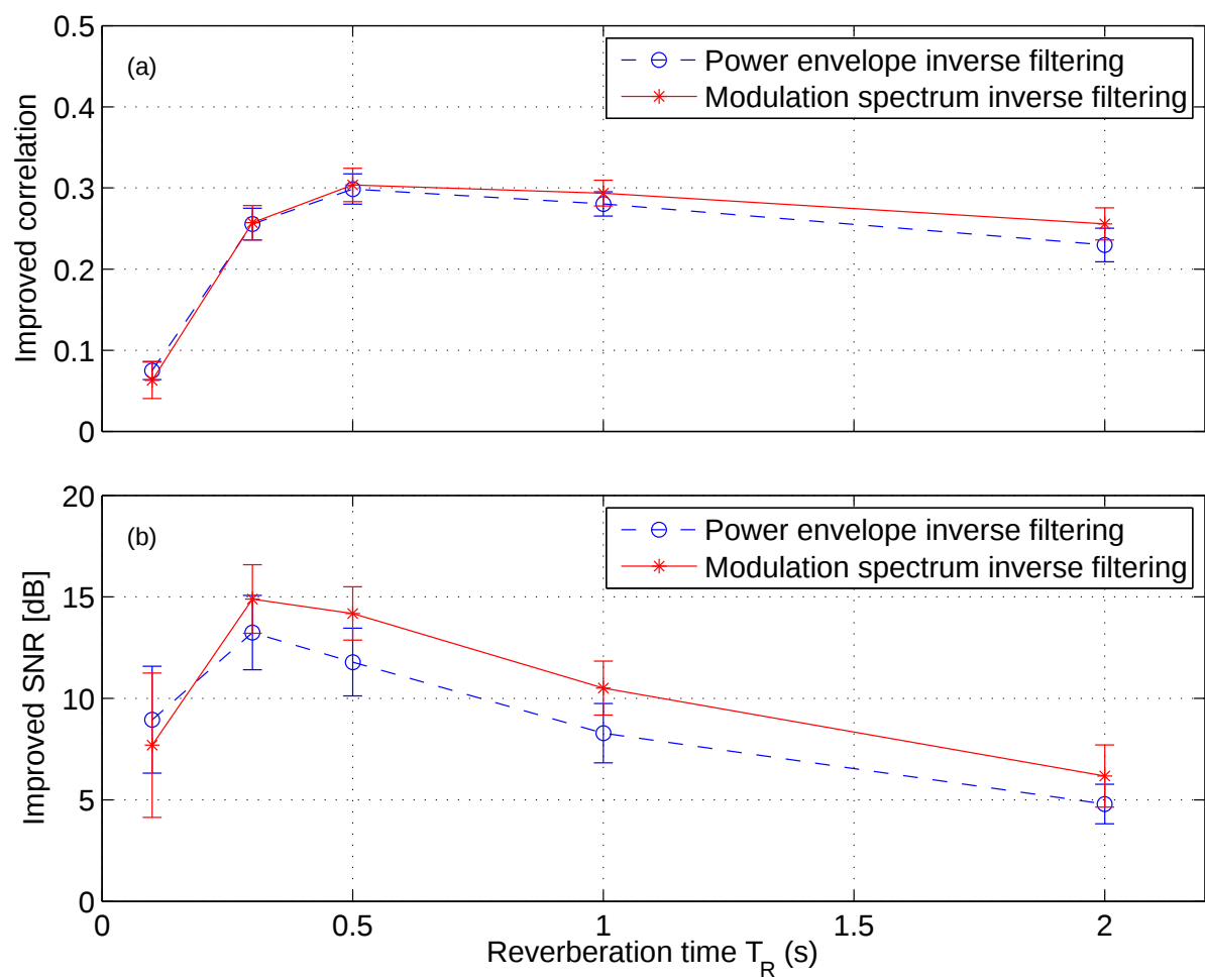
図 6.3: 正弦波で構成されるパワーエンベロープの評価結果：(a) Correlation と (b) SNR の改善度
