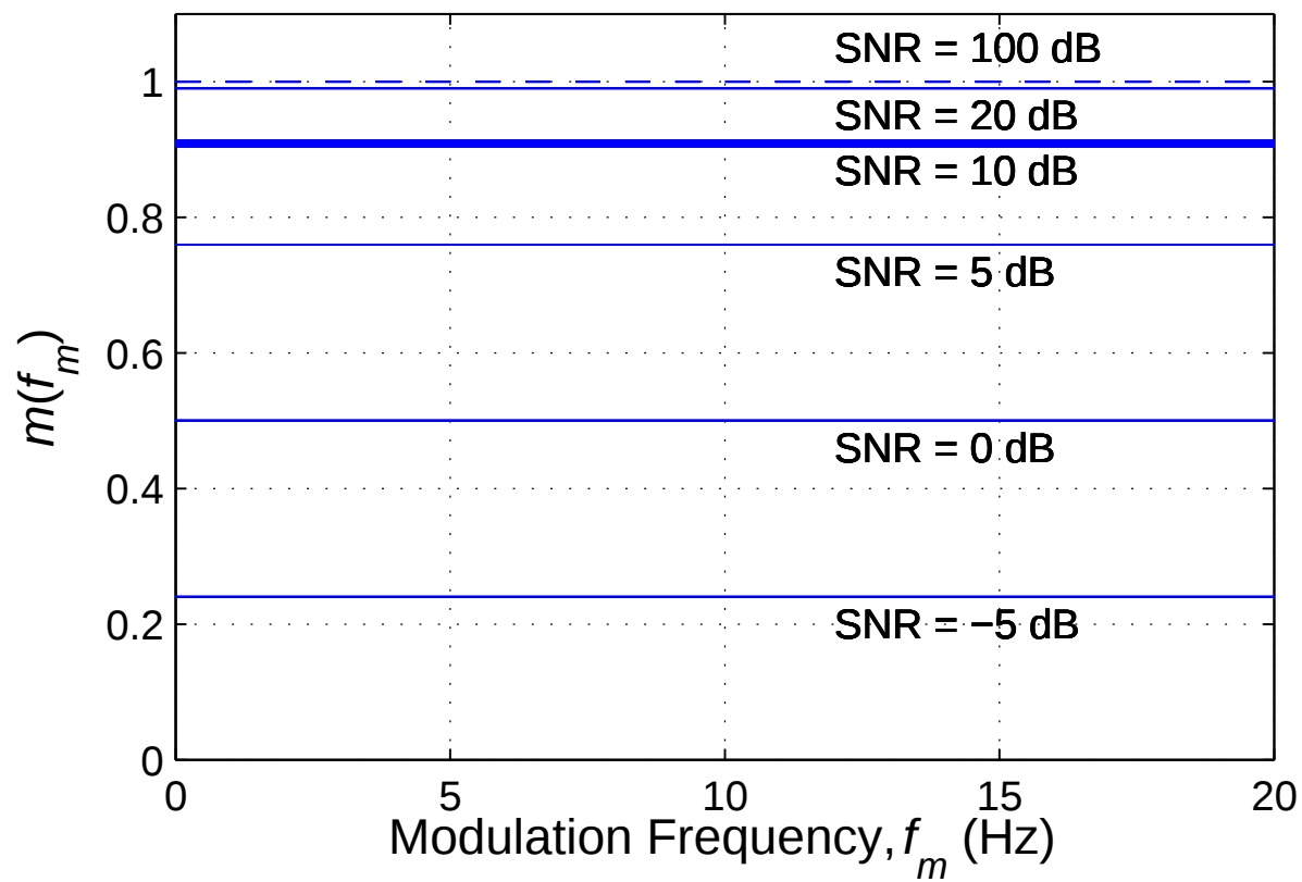
図 4.1: 雑音環境での MTF m(f_m) の特性
