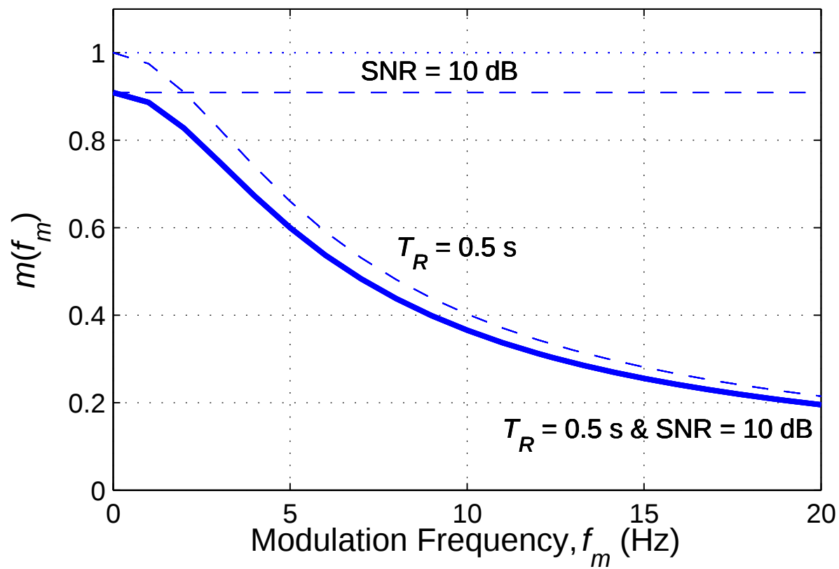
図 4.3: 雑音残響環境での MTF m(f_m) の特性
