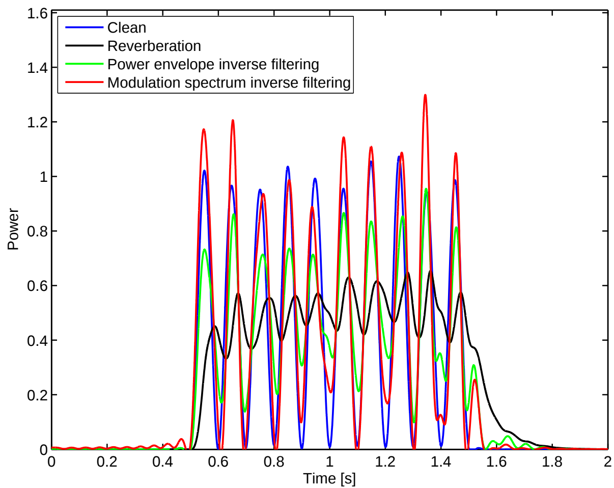
図 6.1: 正弦波信号のパワーエンベロープ
