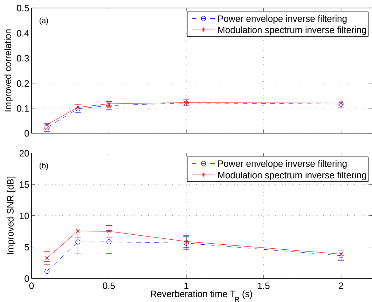
図 6.4: 調波複合音で構成されるパワーエンベロープの評価結果：(a) Correlation と (b) SNR の改善度
