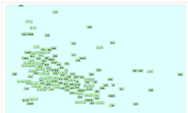
図 3.3: 単語マップ。
