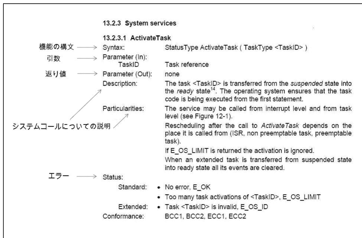
図 2.3: 仕様書の 2 つ目に当たる ActivateTask の章
