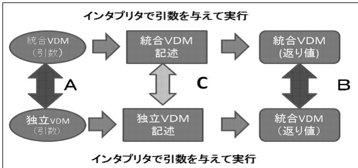
図 5.3: 「独立VDM記述」と「統合VDM記述」の整合性
