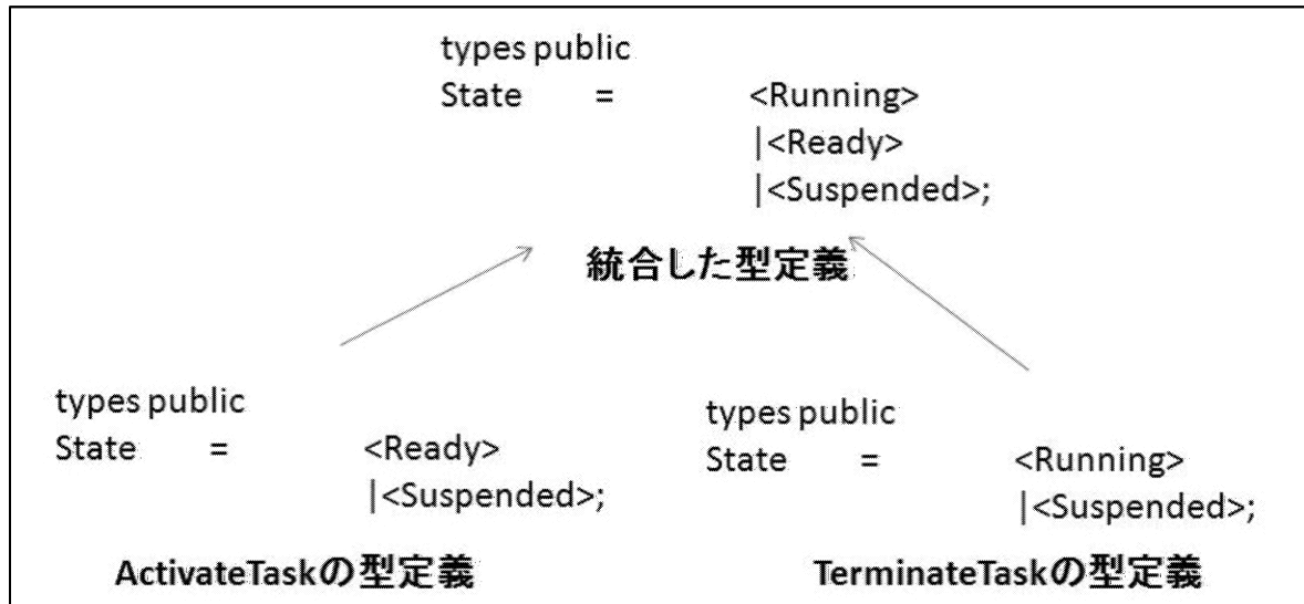
図 3.4: 「統合VDM記述」における型定義の統合
