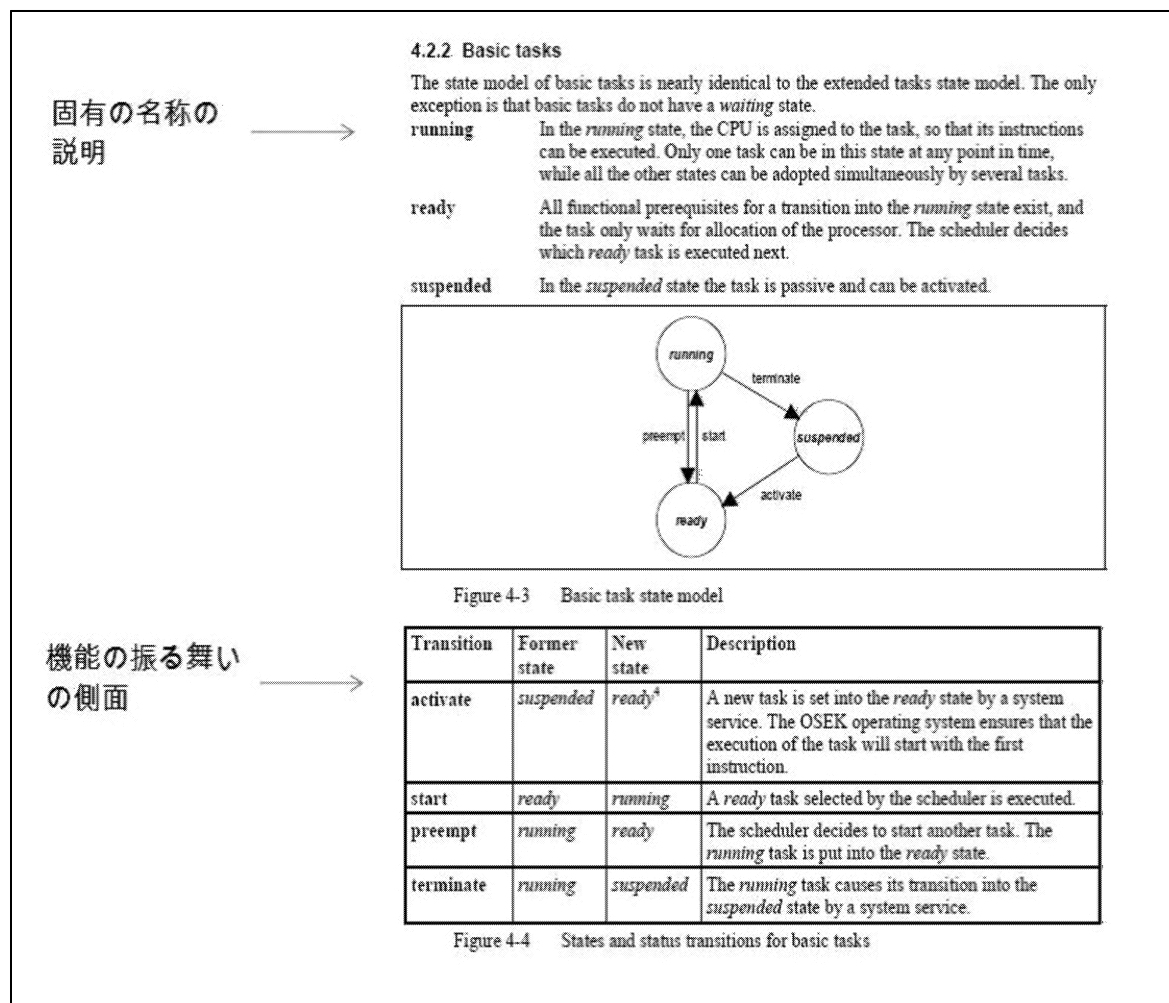
図 2.2: 仕様書の BasicTask の章
