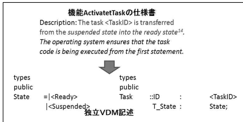
図 3.2: 「独立VDM記述」の型定義の変換
