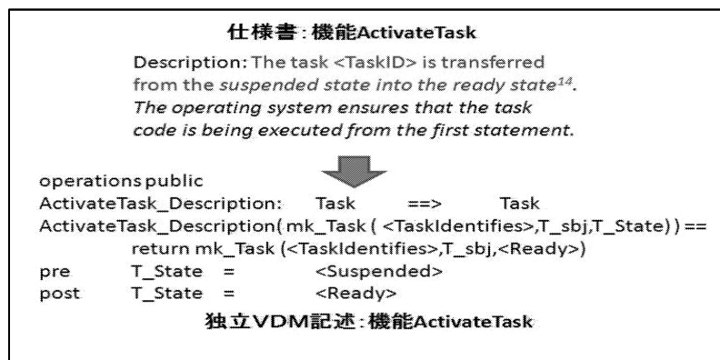
図 3.3: 独立VDM記述: 機能の形式化
