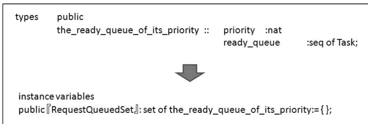
図 3.5: 「統合VDM記述」における型定義から変数の例
