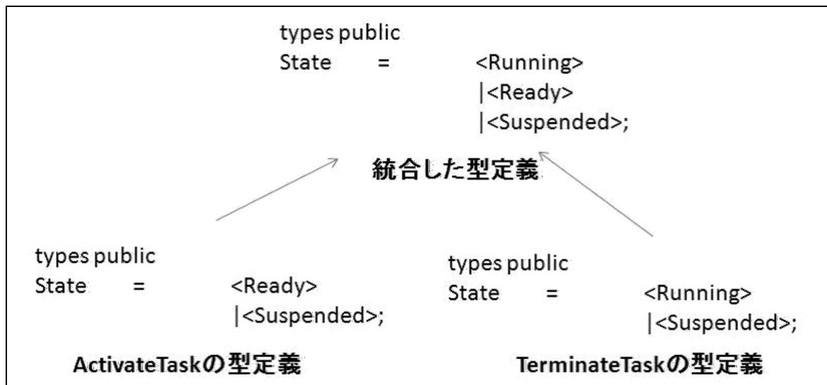
図 5.1: 「統合VDM記述」における型定義の統合
