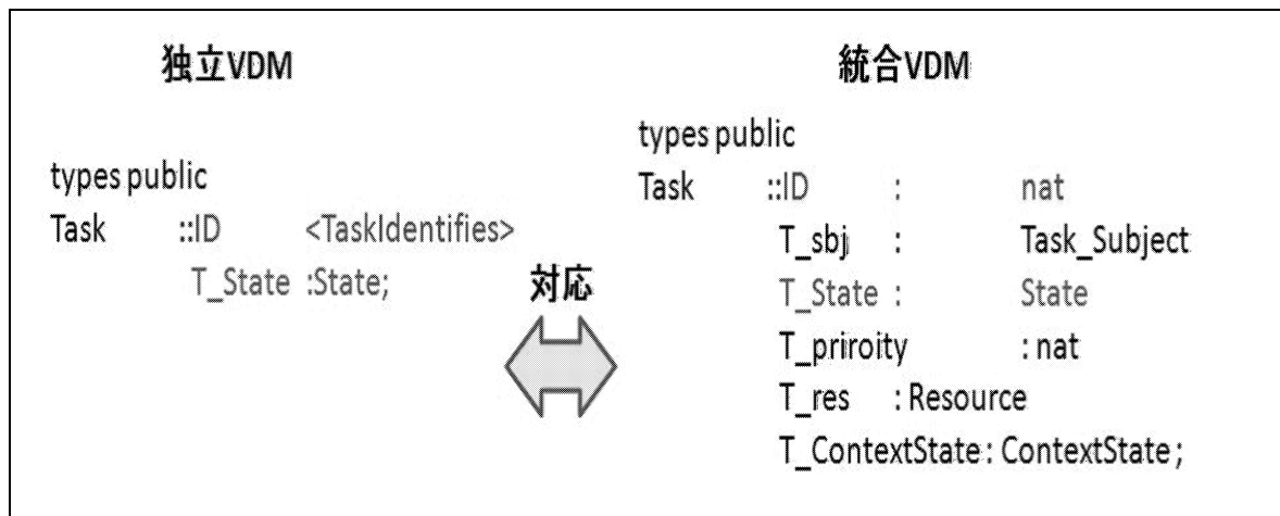
図 5.4: 「独立VDM記述」タスクの型と「統合VDM記述」のタスクの型
