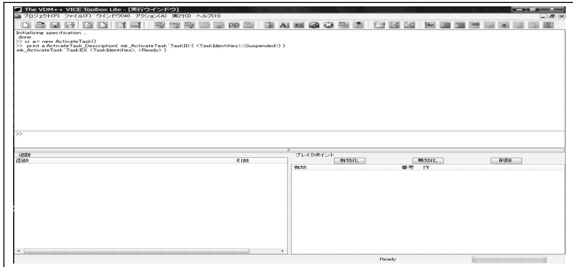
図 2.1: ActivateTask.Description の実行
