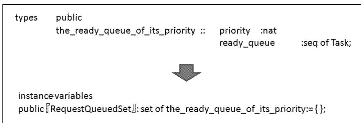
図 5.2: 「統合VDM記述」における型定義から変数の例
