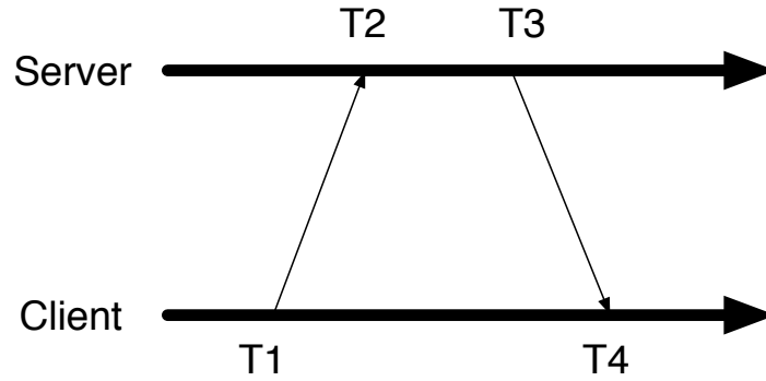
図 5.1: SNTP おける 2-way 時間同期
