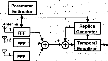
Fig. 1: Optimal S/T-Equalizer
