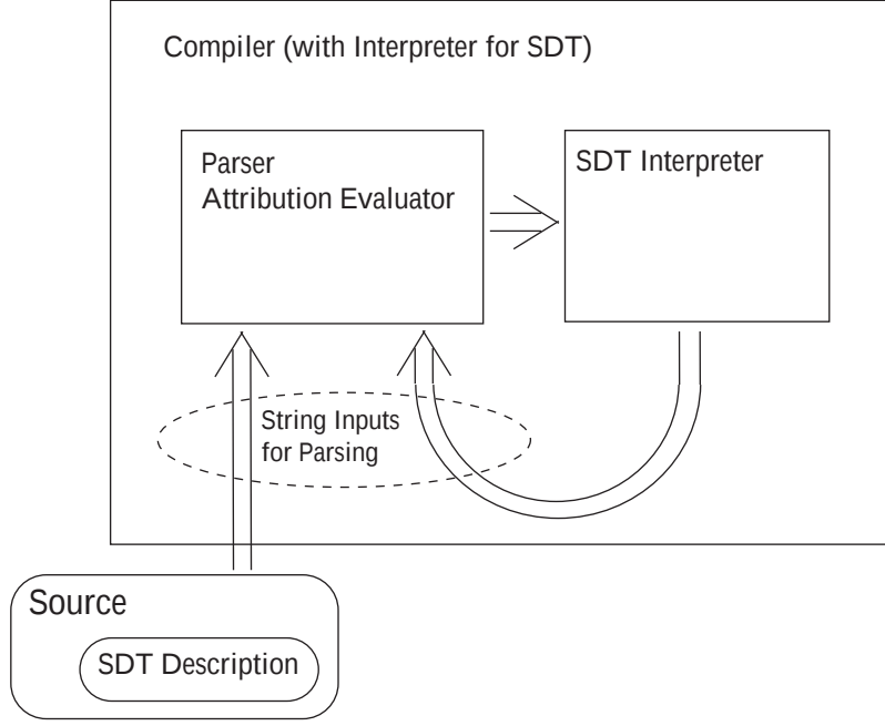
Figure A.4: SDT Interpreter
