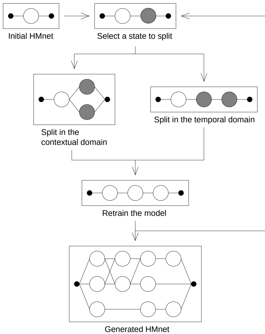
図 C.1: ML-SSS 法の処理の流れ
