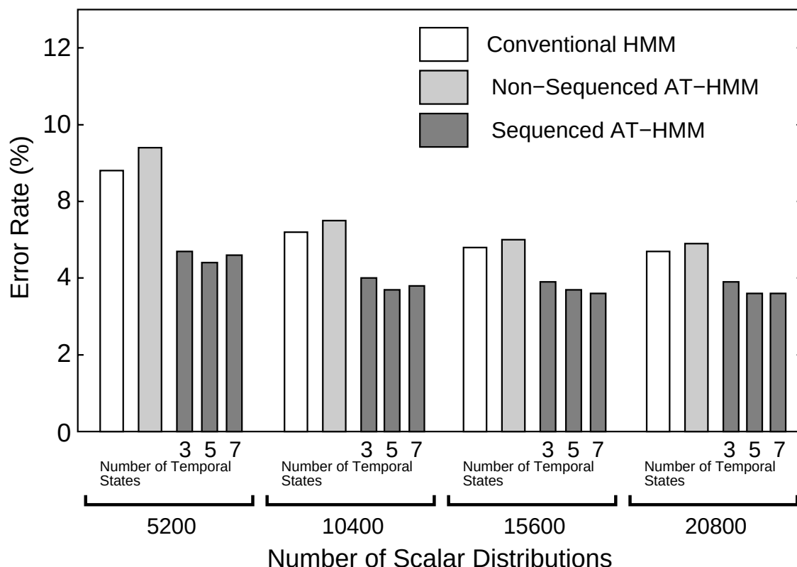
図 3.11: 完全同期な従来型 HMM と順序制約無し/付き AT-HMM の音素誤り率
