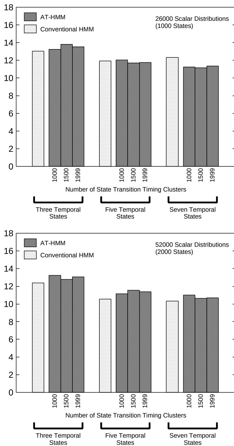
図 3.19: AT-HMM と従来型 HMM の不特定話者連続音素認識実験結果 1
