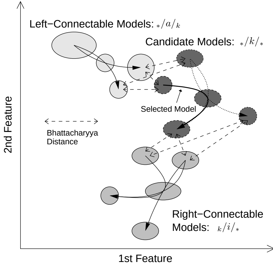
図 B.1: モデル補間法 の概念図
