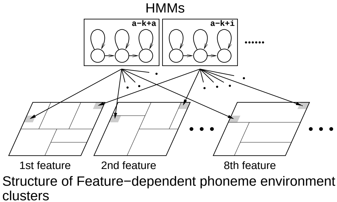
図 4.3: 特徴量依存音素環境クラスタ構造の概念図
