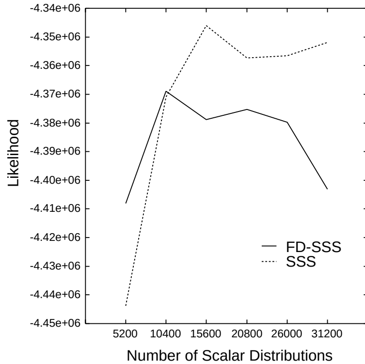
図 4.8: FD-SSS と ML-SSS により生成されたパラメータ共有構造を持つ AT-HMM の評価データに対する尤度
