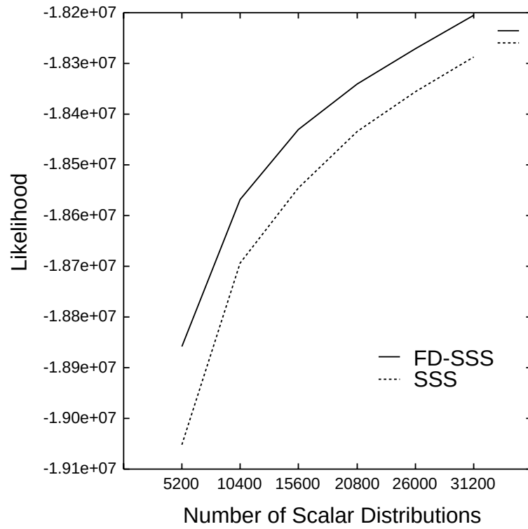
図 4.7: FD-SSS と ML-SSS により生成されたパラメータ共有構造を持つ AT-HMM の学習データに対する尤度
