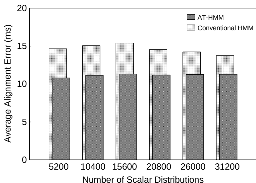
図 3.18: Viterbi セグメンテーションにより計算された音素境界と視察ラベル情報の間の平均誤差
