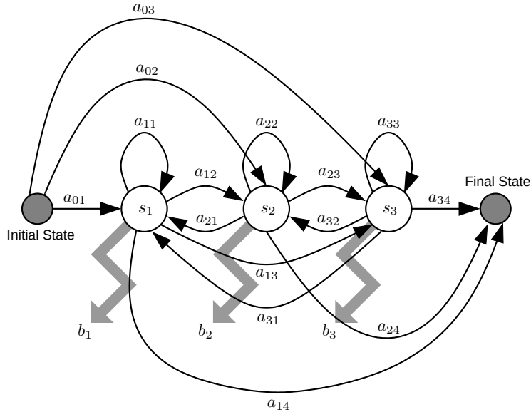
図 2.3: 隠れマルコフモデルの構造
