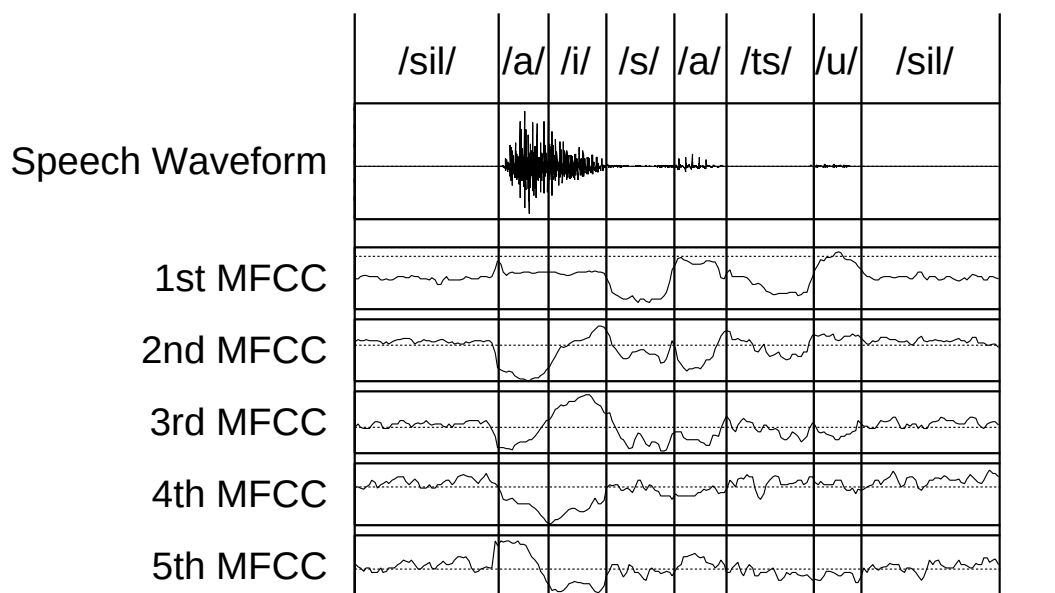
図 2.2: 単語「あいさつ」の音声波形を音響分析することにより得られた，第 1MFCC から第 5MFCC の時間変化
