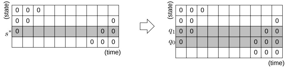
図 C.4: 状態 s から仮状態 q_0 と q_1 への時間方向分割における計算範囲
