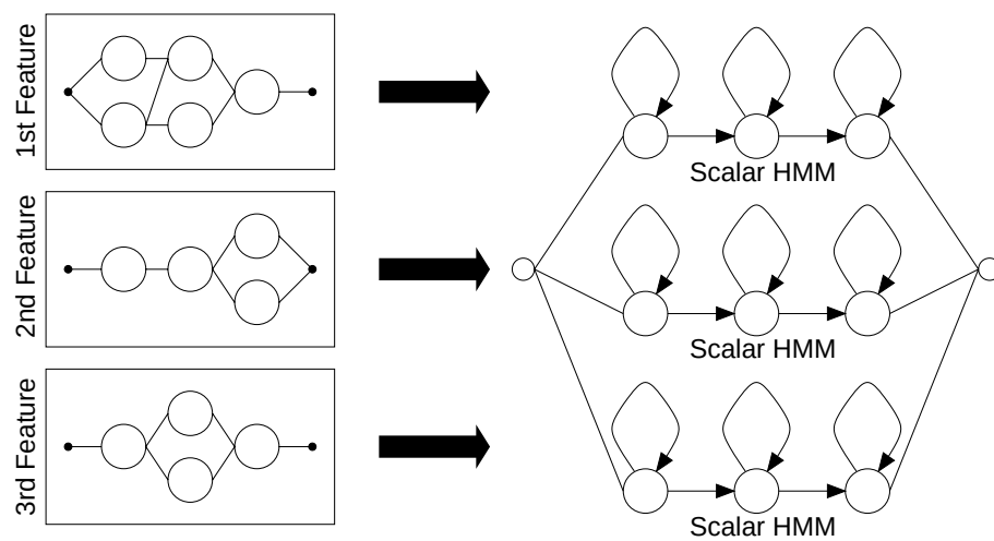
(B) Asynchronous FD-SSS
