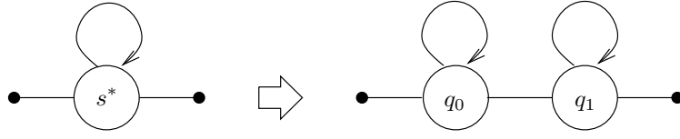
図 C.3: 状態 s^* から状態 q_0 と q_1 への時間方向分割
