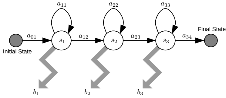
図 2.4: Left-to-right 型隠れマルコフモデルの構造
