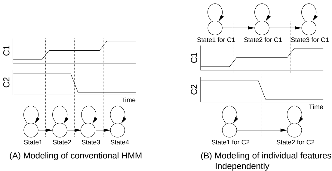
図 3.2: 個々の特徴量が状態遷移に同期して変化する従来の HMM と、個々の特徴量が非同期に状態遷移するモデル
