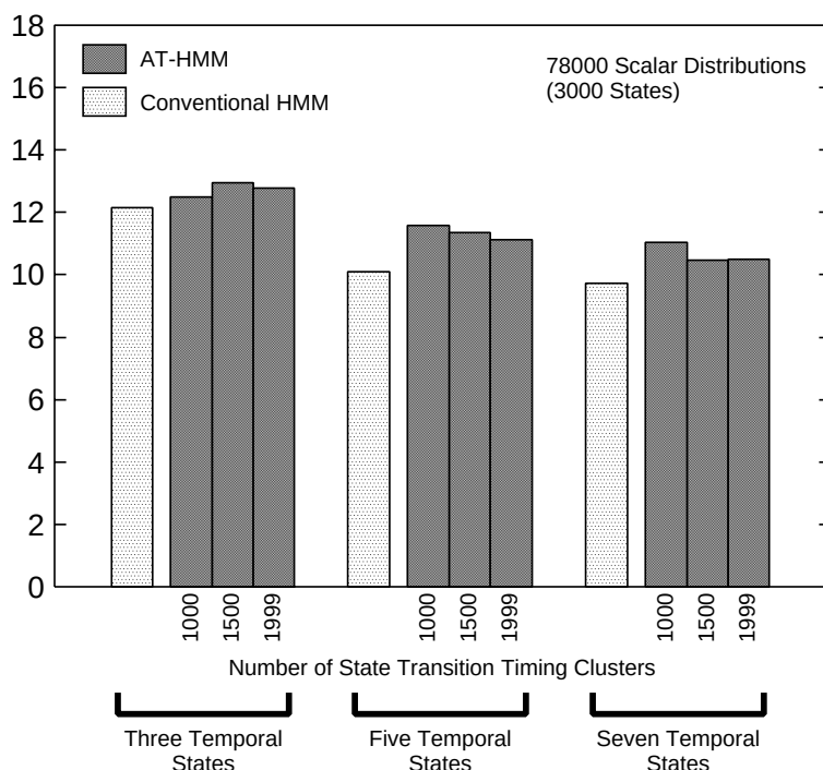
図 3.20: AT-HMM と従来型 HMM の不特定話者連続音素認識実験結果 2
