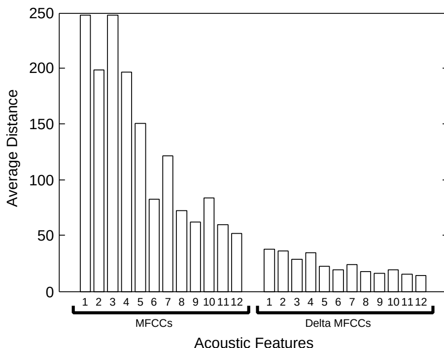
図 4.1: 1000 状態 8 混合の HMM における個々の特徴量の分布間平均距離
