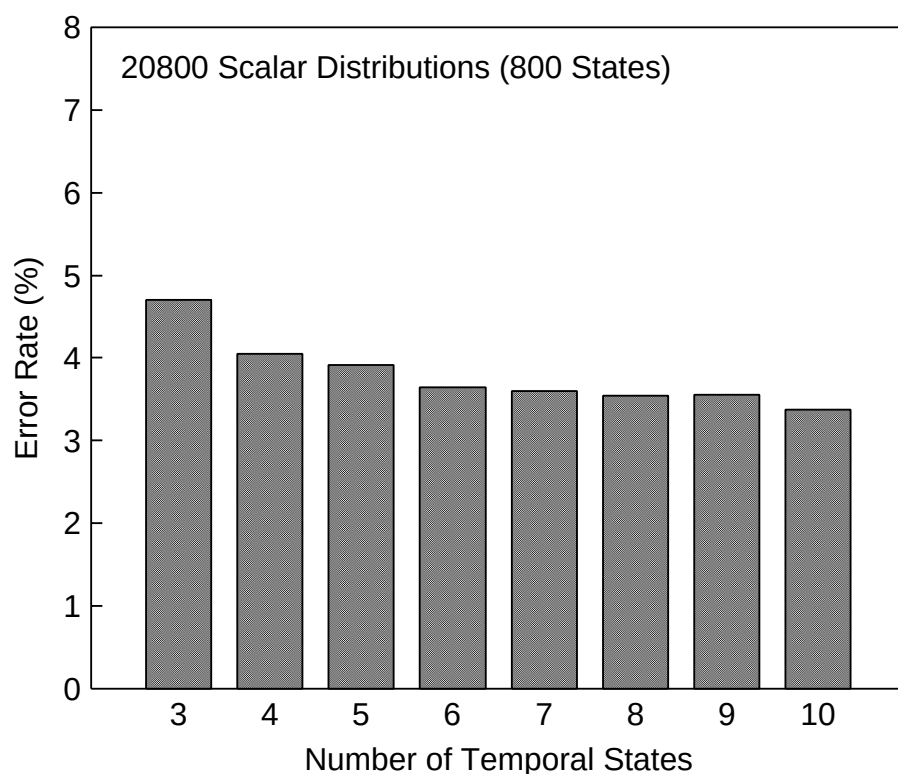
図 3.10: 種々の時間方向状態数を持つ順序制約付き AT-HMM の音素誤り率
