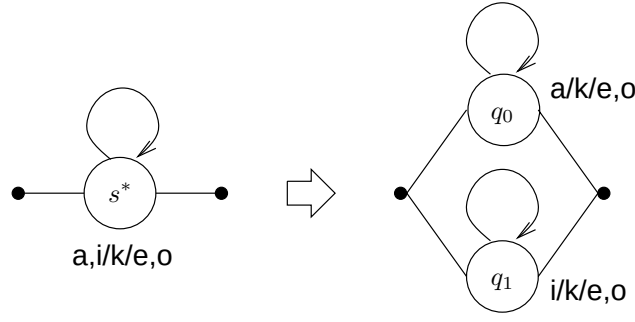
図 C.2: 状態 s^* から状態 q_0 と q_1 への先行音素環境要因による音素環境方向分割
