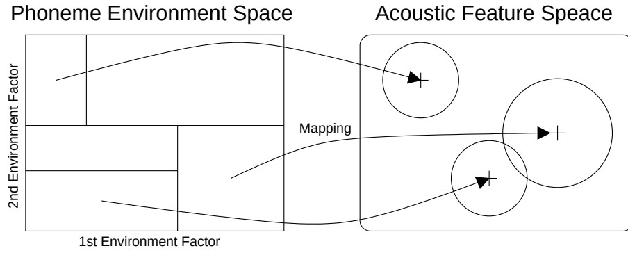
図 4.2: 音素環境空間と音響特徴量空間の間の写像関係の概念図
