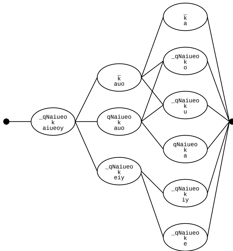
図 C.5: ML-SSS により生成された音素/k/の HMnet
