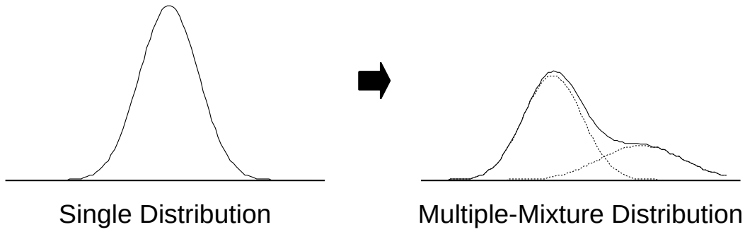
図 2.5: 複数混合分布化による状態出力確率分布の精密化
