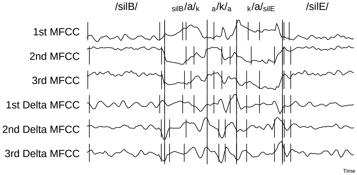
図 3.16: 順序制約付き AT-HMM による単語「赤」/aka/に対する Viterbi セグメンテーション結果
