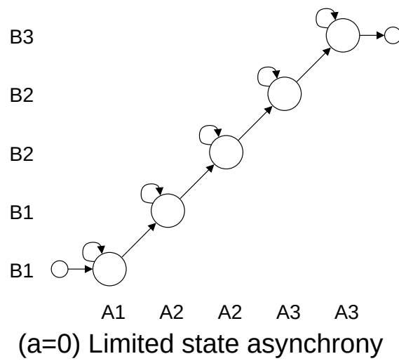
図 3.6: 順順序制約付き AT-HMM の実現 (a は時間ずれ状態数を表す)
