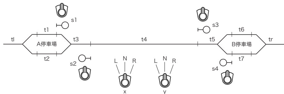
図 6.1: 二隣接駅の鉄道システム
