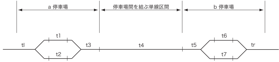
図 3.1: スタッフ閉そくを適用した鉄道システム
