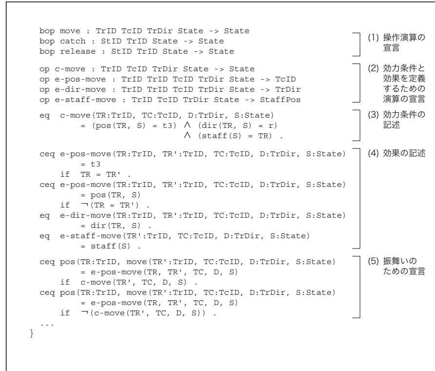
図 3.4: モジュール STAFFSYSTEM
