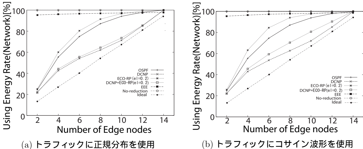
図 5.6.2: NSFNET T1(乱数コスト使用時) の平均消費電力
