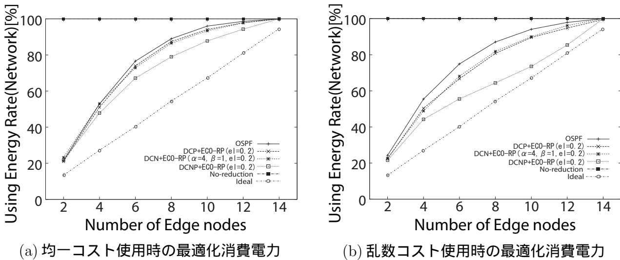
図 5.4.1: NSFNET T1 の消費電力
