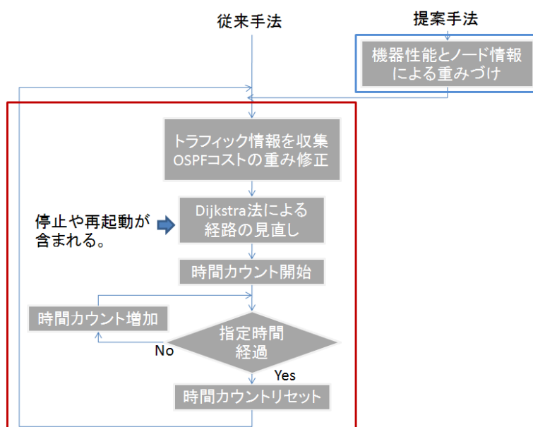
図 4.2.1: 従来手法と提案手法
