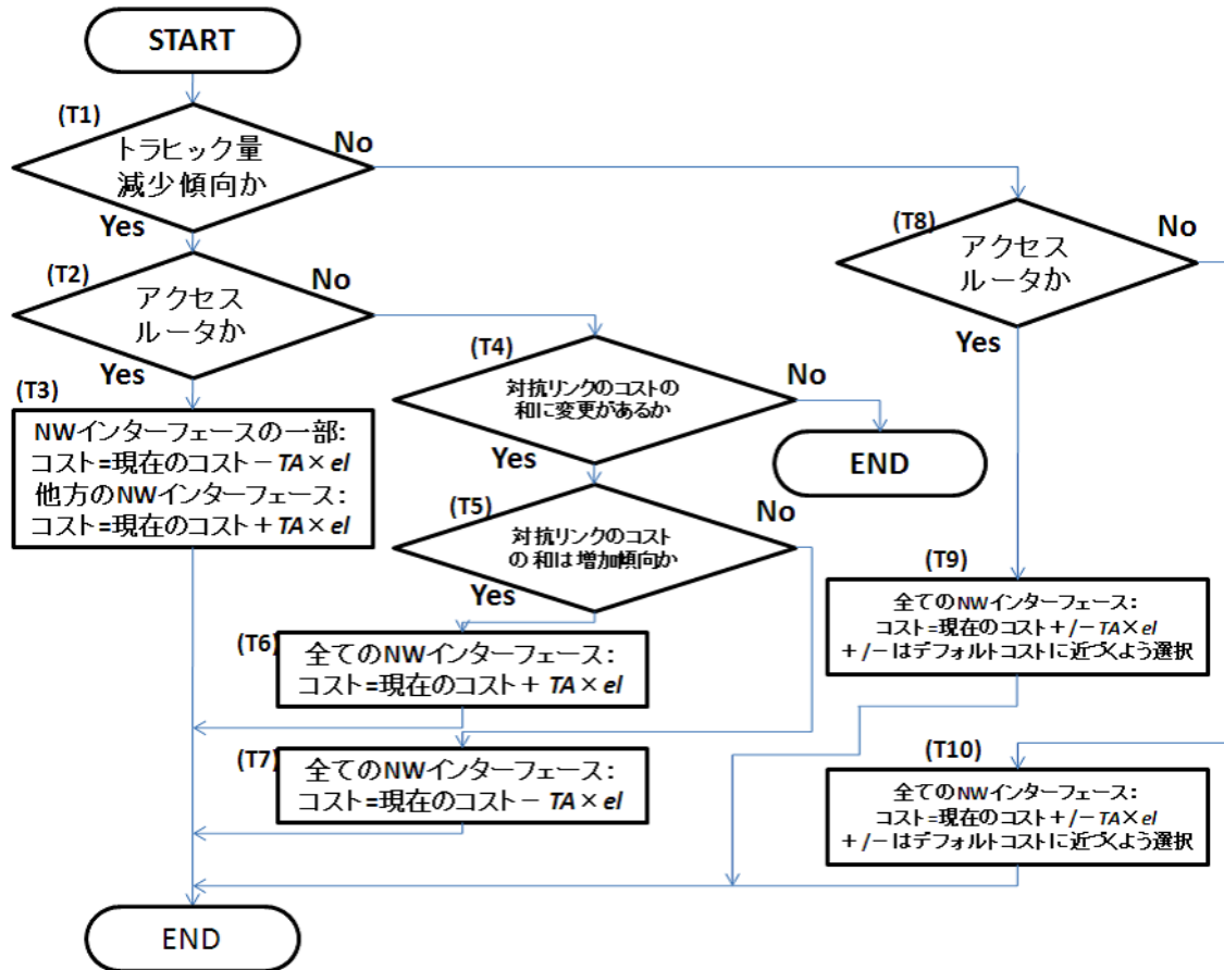
図 2.3.4: 荒井らが提案した ECO-RP の動的 OSPF コスト更新 [12]
