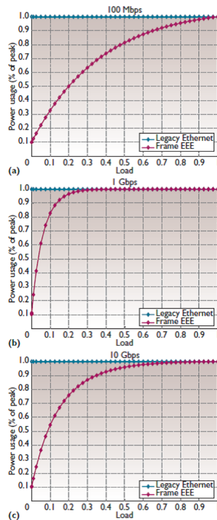
図 2.2.2: Reviriego らが使用した EEE の消費電力表 [8]
