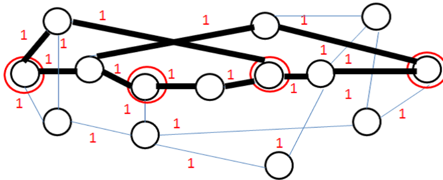
図 2.3.2: Dijkstra 法によるルーティング (黒太線)
