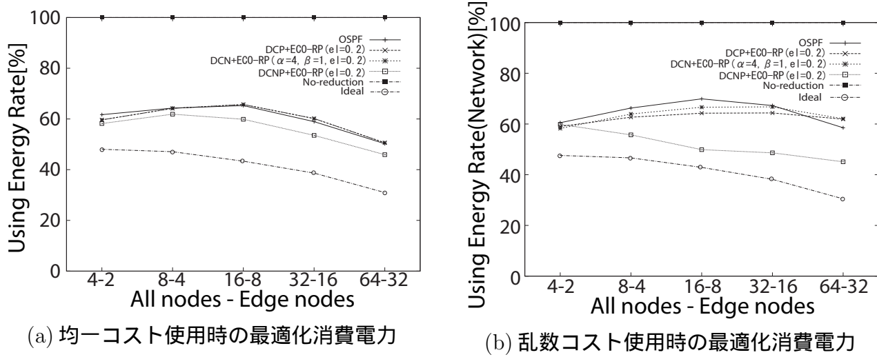
図 5.4.2: ランダム生成ネットワークの消費電力
