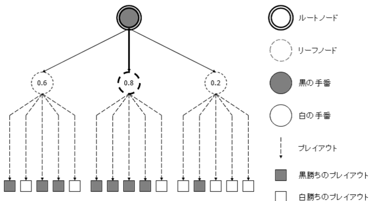
図 2.2 原始モンテカルロ囲碁の評価の例
