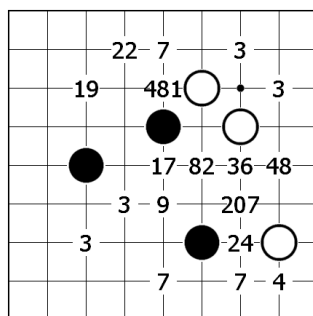
(b) 6 手進んだ局面（黒番）
