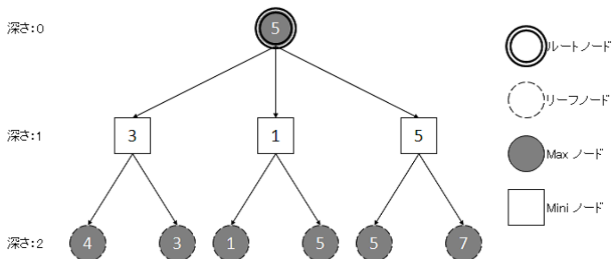
図 2.3 Minmax アルゴリズムの評価の例
