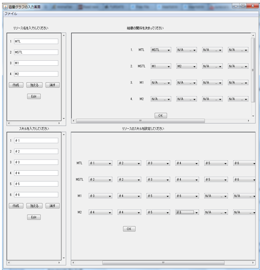
図 4.4 LCB プロトタイプ の容量グラフ入力画面
